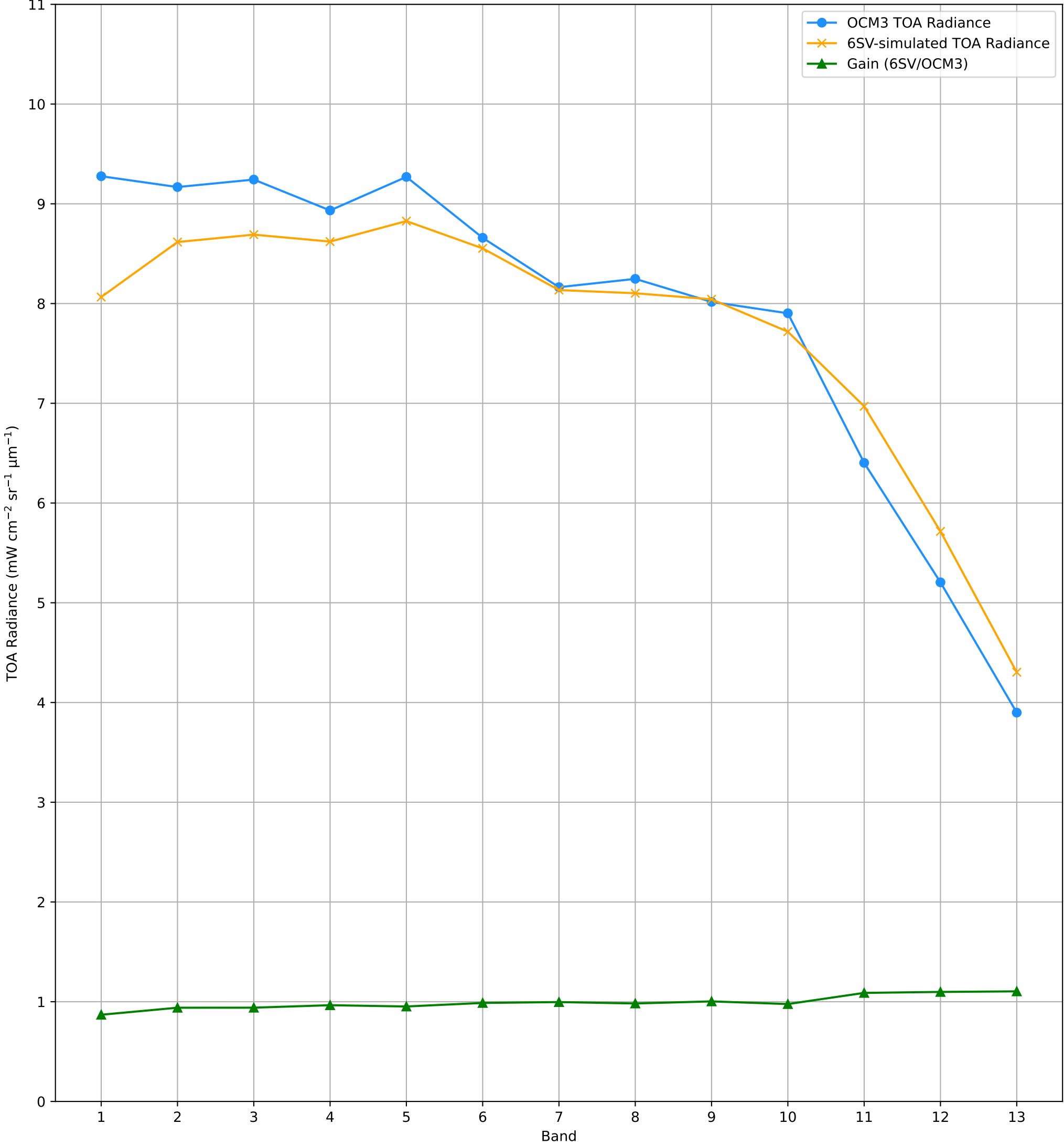
TOA Radiance (OCM3 vs. 6SV) over RVUS RadCalNet Site Lat: 38.497°, Lon: -115.69° - 09-JAN-2026 (STRIP_ID: 16495)
