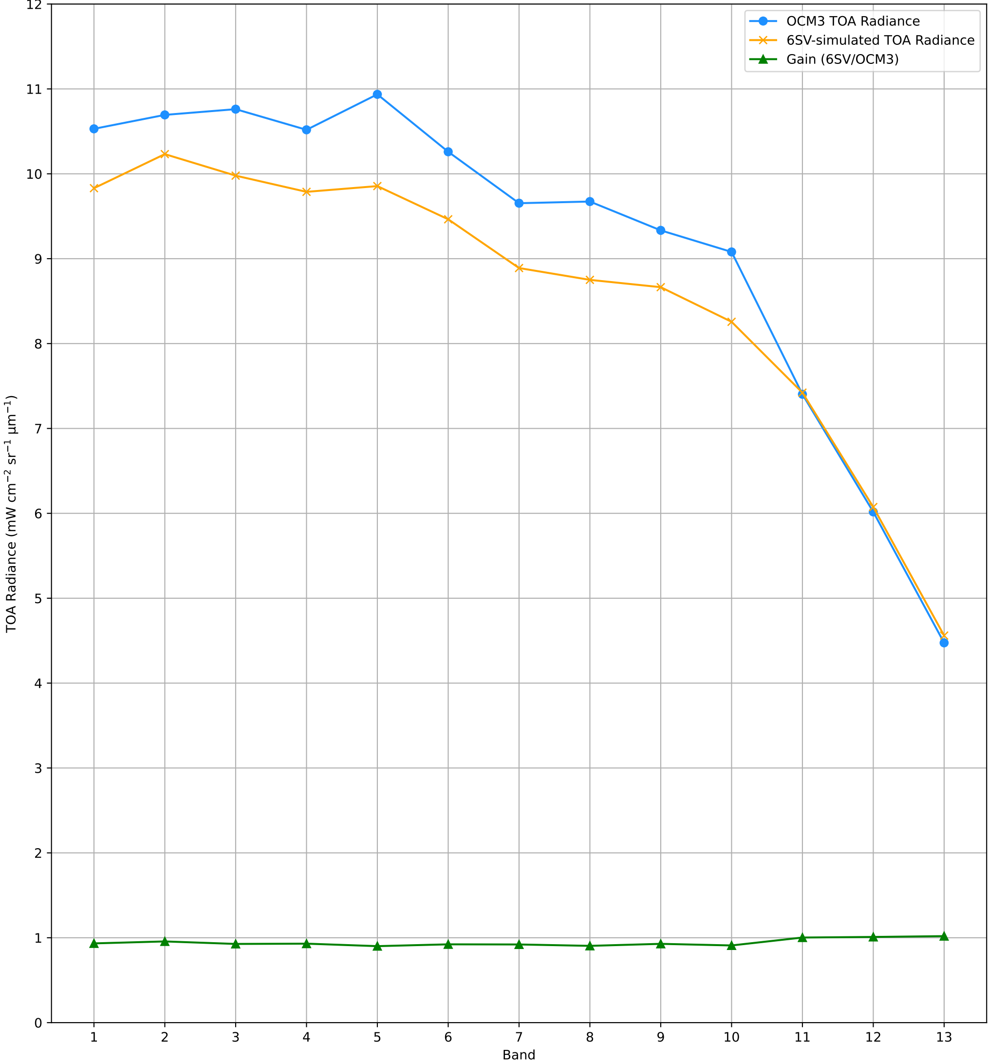
TOA Radiance (OCM3 vs. 6SV) over RVUS RadCalNet Site Lat: 38.497°, Lon: -115.69° - 14-JAN-2026 (STRIP_ID: 16567)
