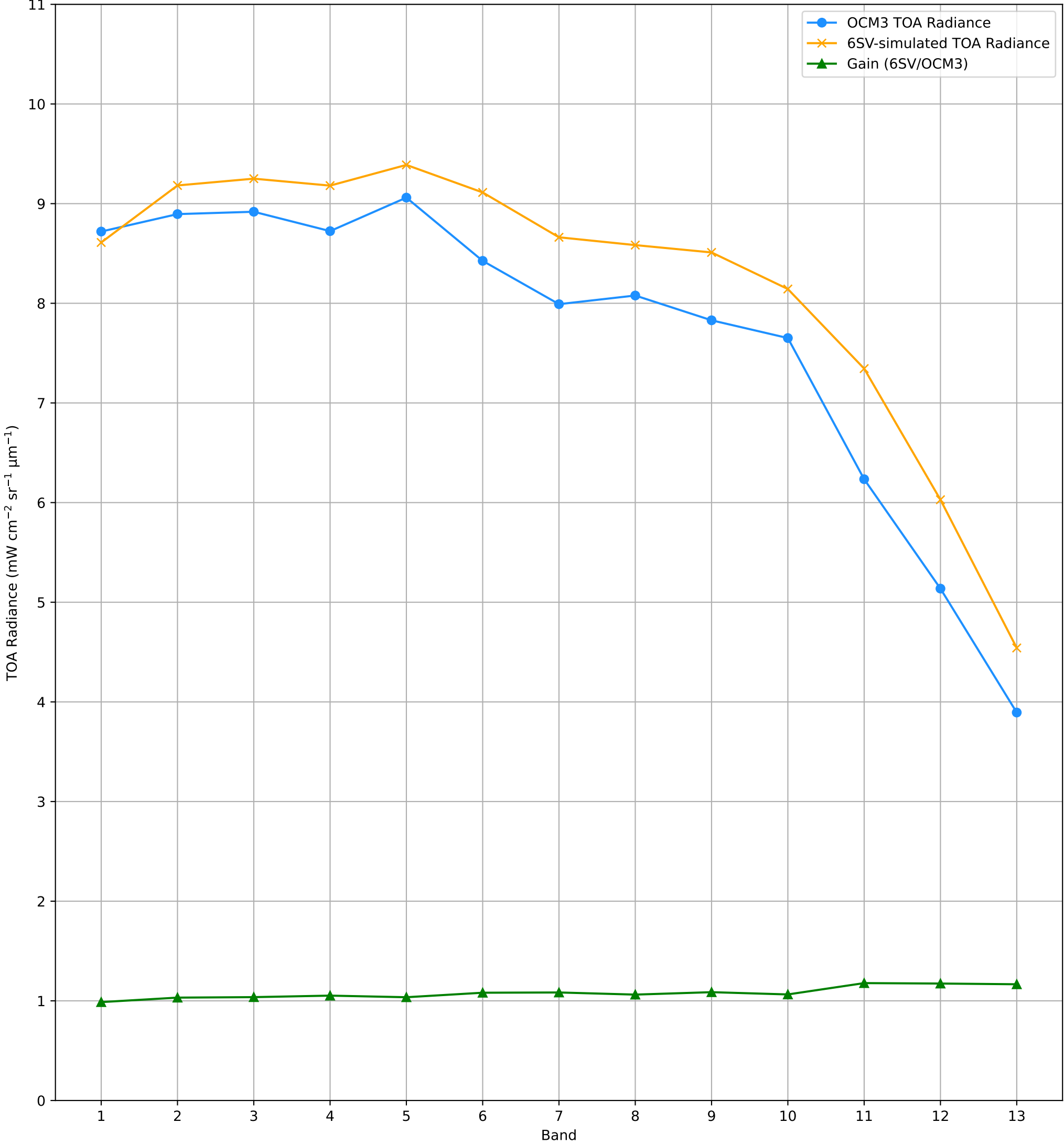
TOA Radiance (OCM3 vs. 6SV) over RVUS RadCalNet Site Lat: 38.497°, Lon: -115.69° - 17-JAN-2026 (STRIP_ID: 16611)
