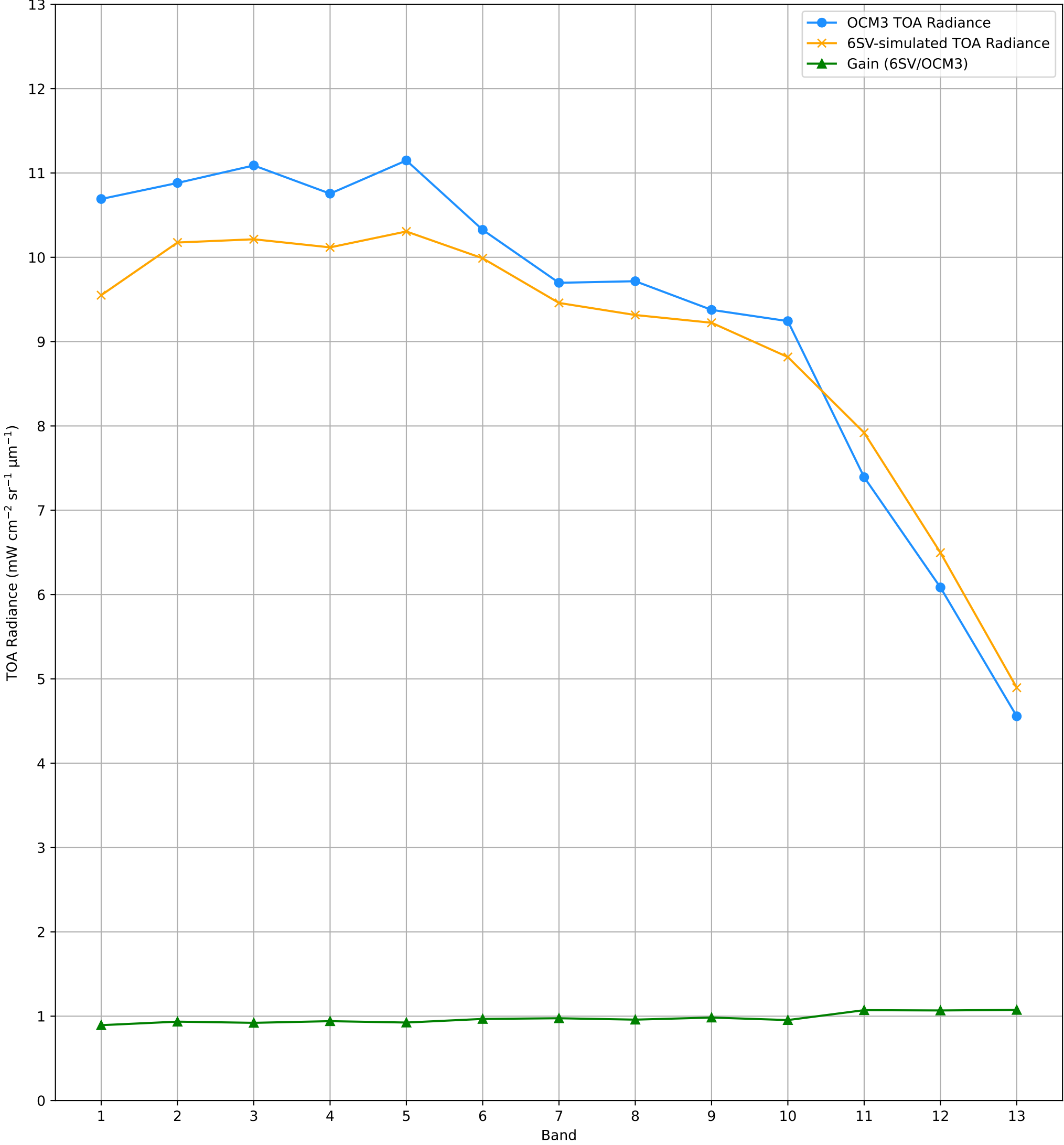
TOA Radiance (OCM3 vs. 6SV) over RVUS RadCalNet Site Lat: 38.497°, Lon: -115.69° - 18-JAN-2026 (STRIP_ID: 16625)
