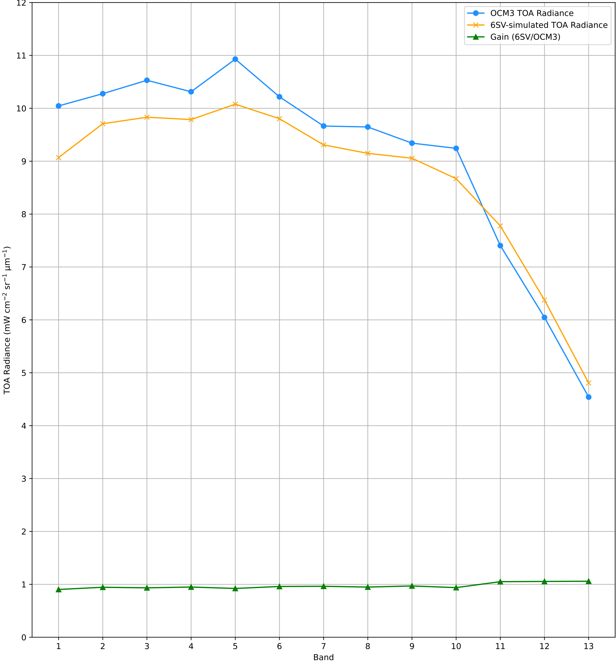
TOA Radiance (OCM3 vs. 6SV) over RVUS RadCalNet Site Lat: 38.497°, Lon: -115.69° - 20-JAN-2026 (STRIP_ID: 16654)
