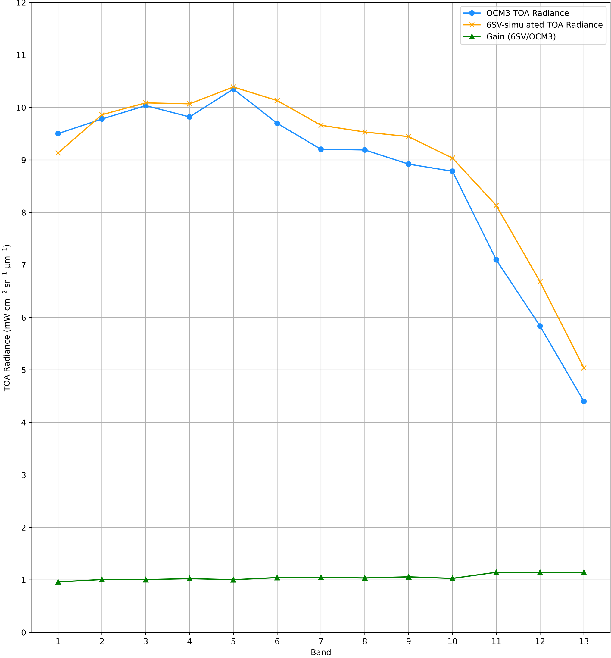
TOA Radiance (OCM3 vs. 6SV) over RVUS RadCalNet Site Lat: 38.497°, Lon: -115.69° - 28-JAN-2026 (STRIP_ID: 16770)
