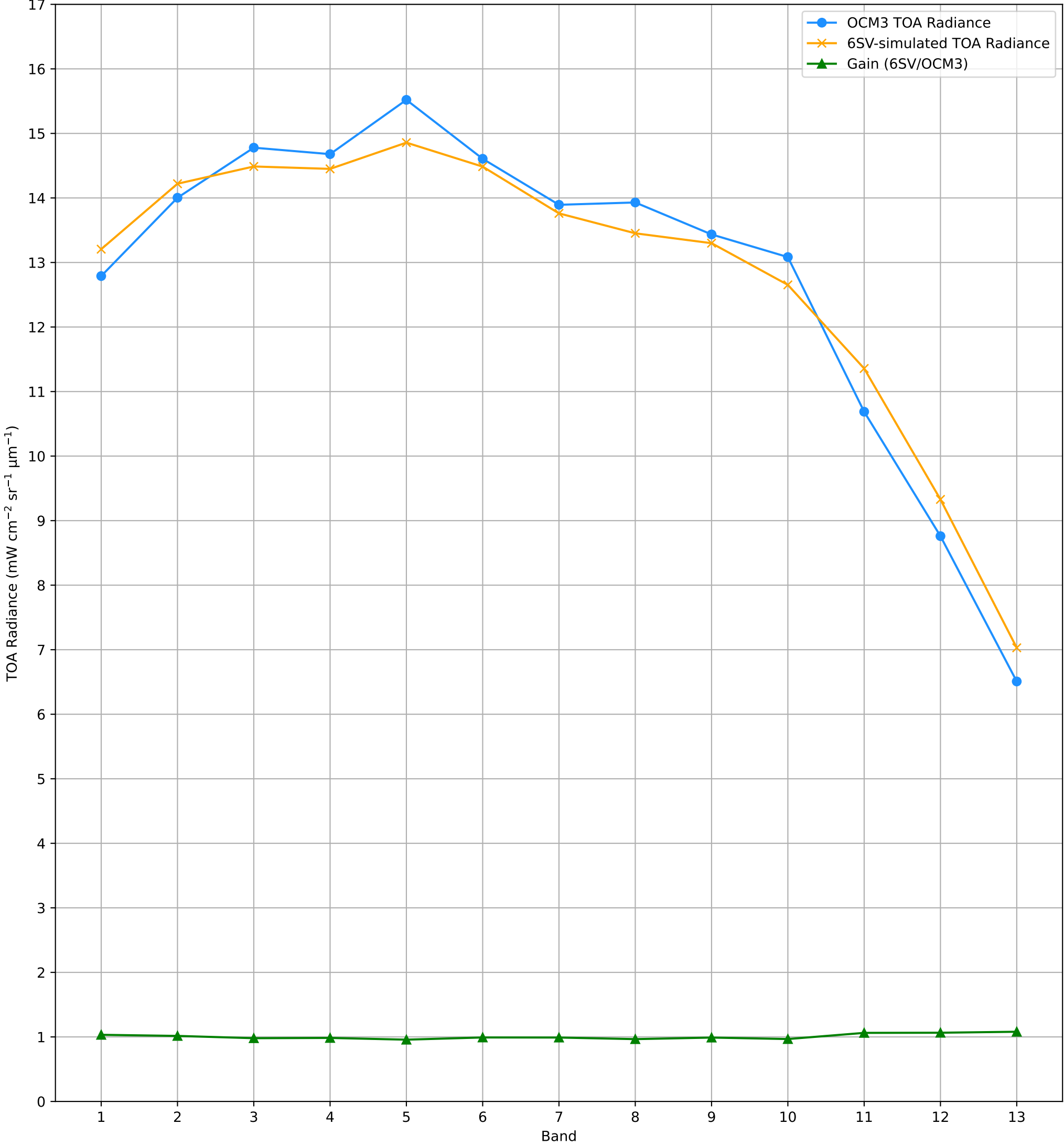
TOA Radiance (OCM3 vs. 6SV) over RVUS RadCalNet Site Lat: 38.497°, Lon: -115.69° - 07-MAR-2026 (STRIP_ID: 17319)
