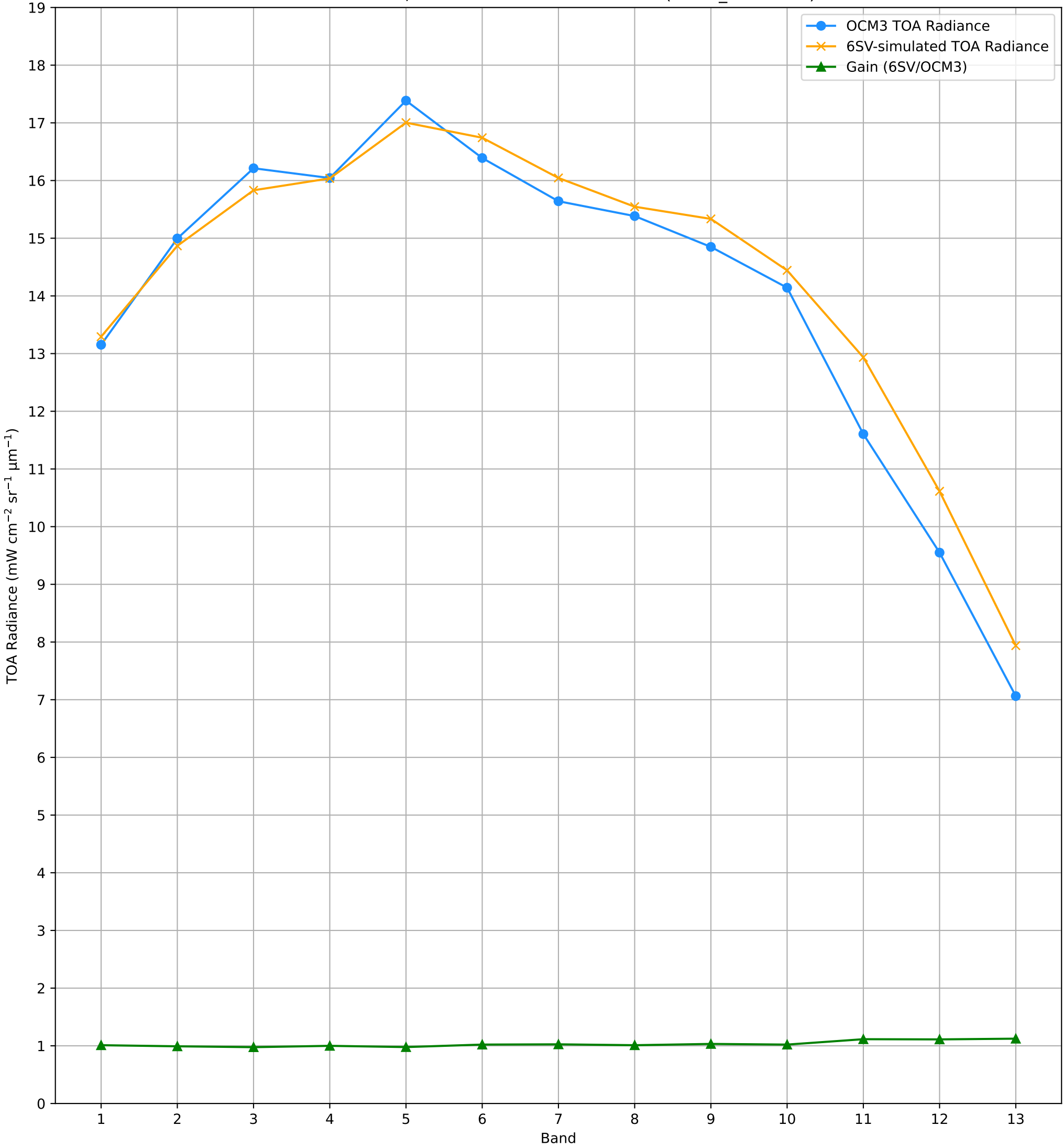
TOA Radiance (OCM3 vs. 6SV) over RVUS RadCalNet Site Lat: 38.497°, Lon: -115.69° - 24-MAR-2026 (STRIP_ID: 17565)
