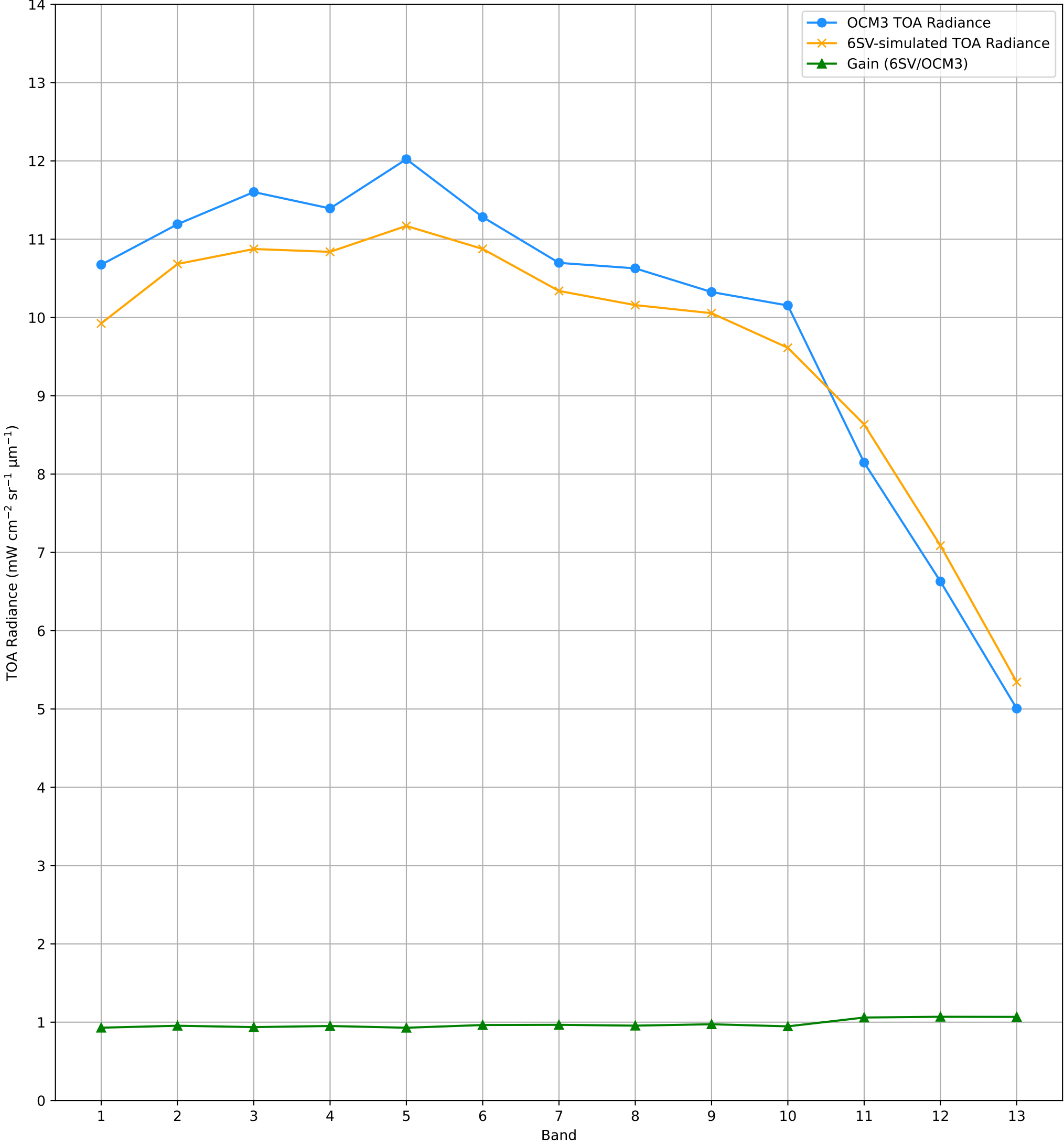
TOA Radiance (OCM3 vs. 6SV) over RVUS RadCalNet Site Lat: 38.497°, Lon: -115.69° - 02-FEB-2026 (STRIP_ID: 16842)
