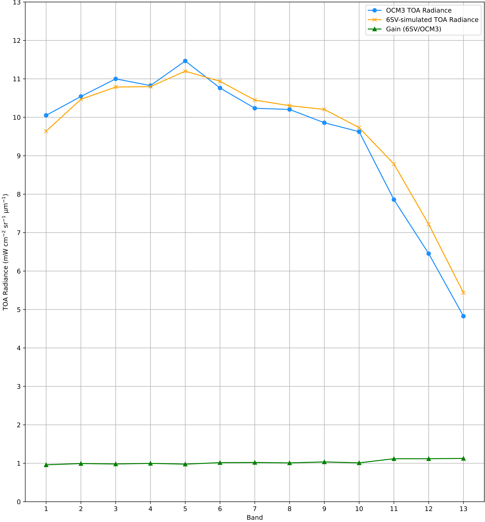
TOA Radiance (OCM3 vs. 6SV) over RVUS RadCalNet Site Lat: 38.497°, Lon: -115.69° - 08-FEB-2026 (STRIP_ID: 16929)
