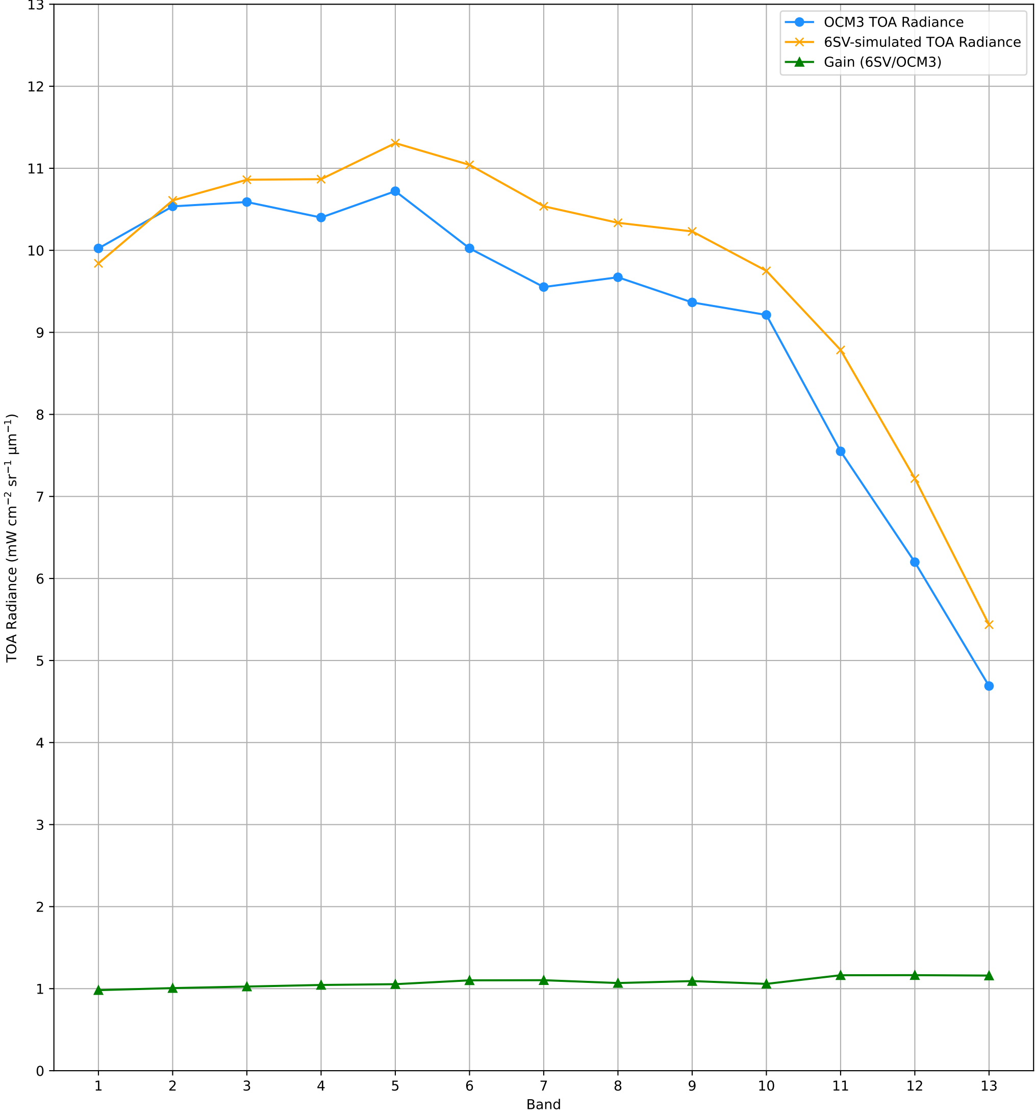
TOA Radiance (OCM3 vs. 6SV) over RVUS RadCalNet Site Lat: 38.497°, Lon: -115.69° - 12-FEB-2026 (STRIP_ID: 16987)
