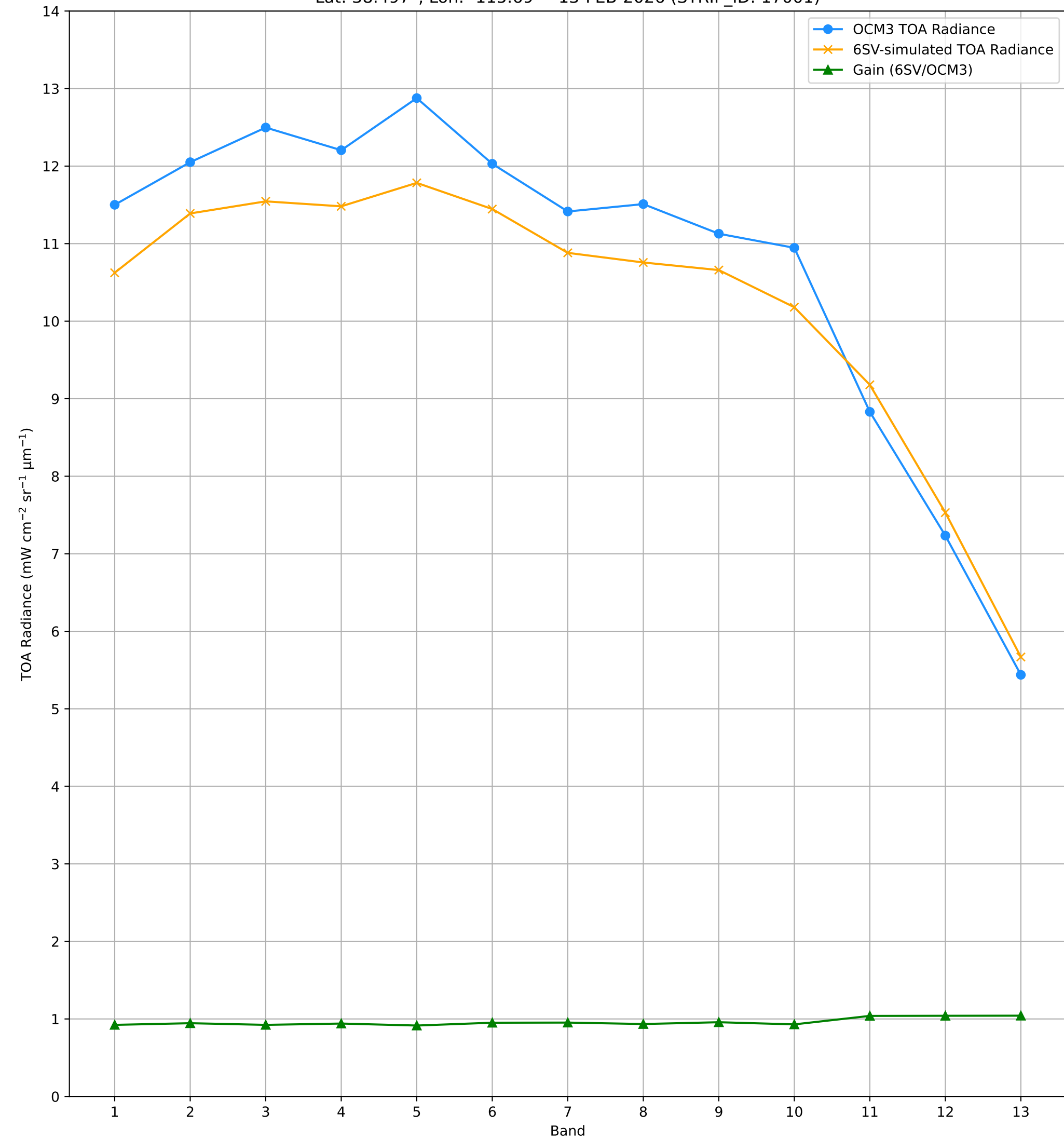
TOA Radiance (OCM3 vs. 6SV) over RVUS RadCalNet Site Lat: 38.497°, Lon: -115.69° - 13-FEB-2026 (STRIP_ID: 17001)
