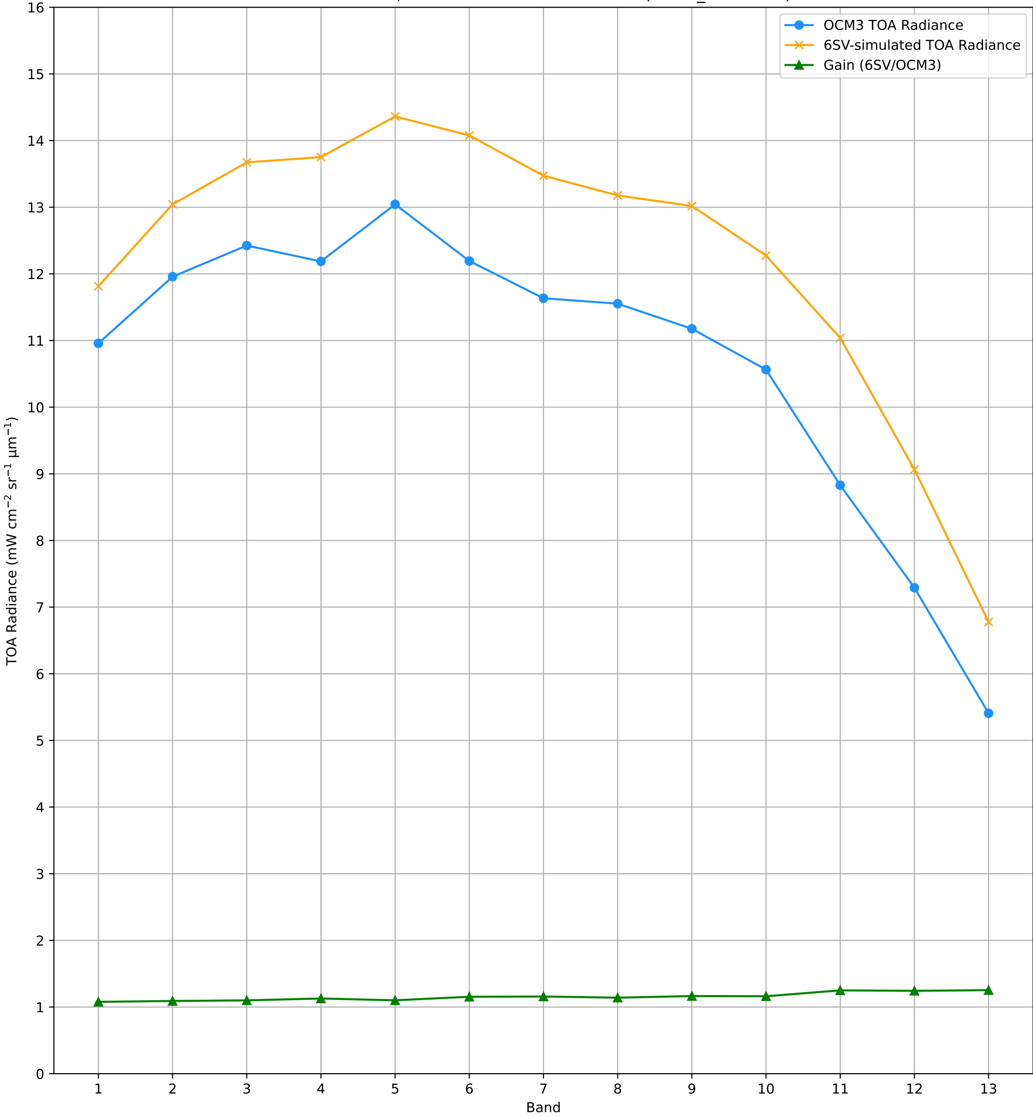
TOA Radiance (OCM3 vs. 6SV) over RVUS RadCalNet Site Lat: 38.497°, Lon: -115.69° - 27-FEB-2026 (STRIP_ID: 17204)
