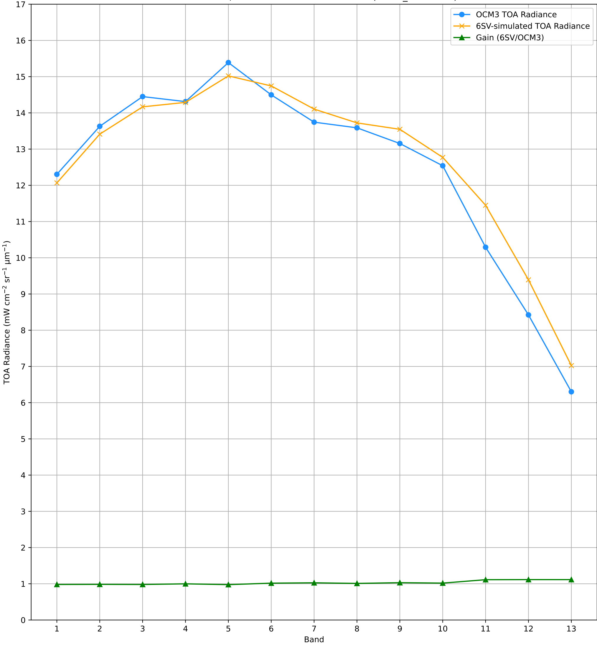
TOA Radiance (OCM3 vs. 6SV) over RVUS RadCalNet Site Lat: 38.497°, Lon: -115.69° - 28-FEB-2026 (STRIP_ID: 17218)
