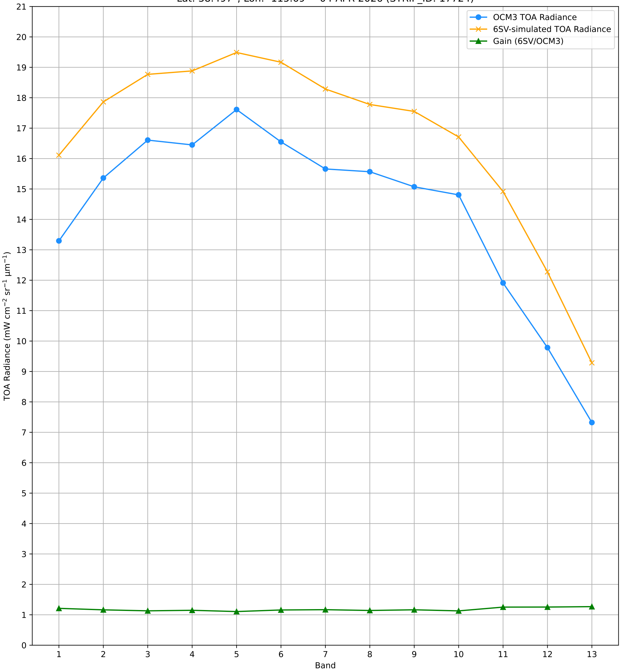
TOA Radiance (OCM3 vs. 6SV) over RVUS RadCalNet Site Lat: 38.497°, Lon: -115.69° - 04-APR-2026 (STRIP_ID: 17724)
