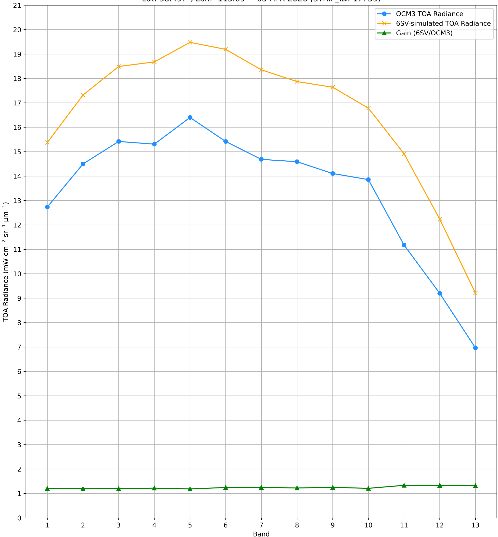
TOA Radiance (OCM3 vs. 6SV) over RVUS RadCalNet Site Lat: 38.497°, Lon: -115.69° - 05-APR-2026 (STRIP_ID: 17739)
