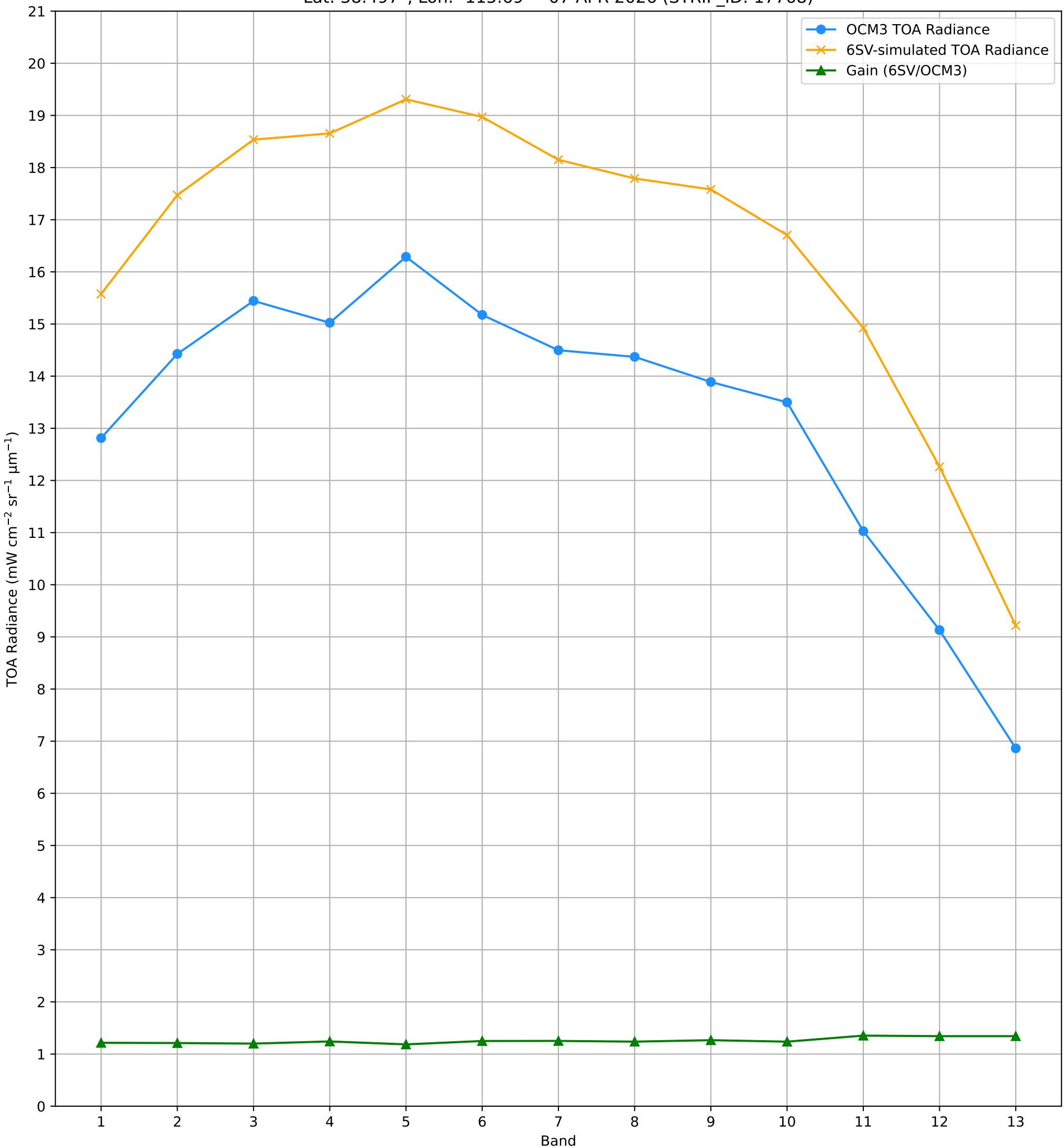
TOA Radiance (OCM3 vs. 6SV) over RVUS RadCalNet Site Lat: 38.497°, Lon: -115.69° - 07-APR-2026 (STRIP_ID: 17768)
