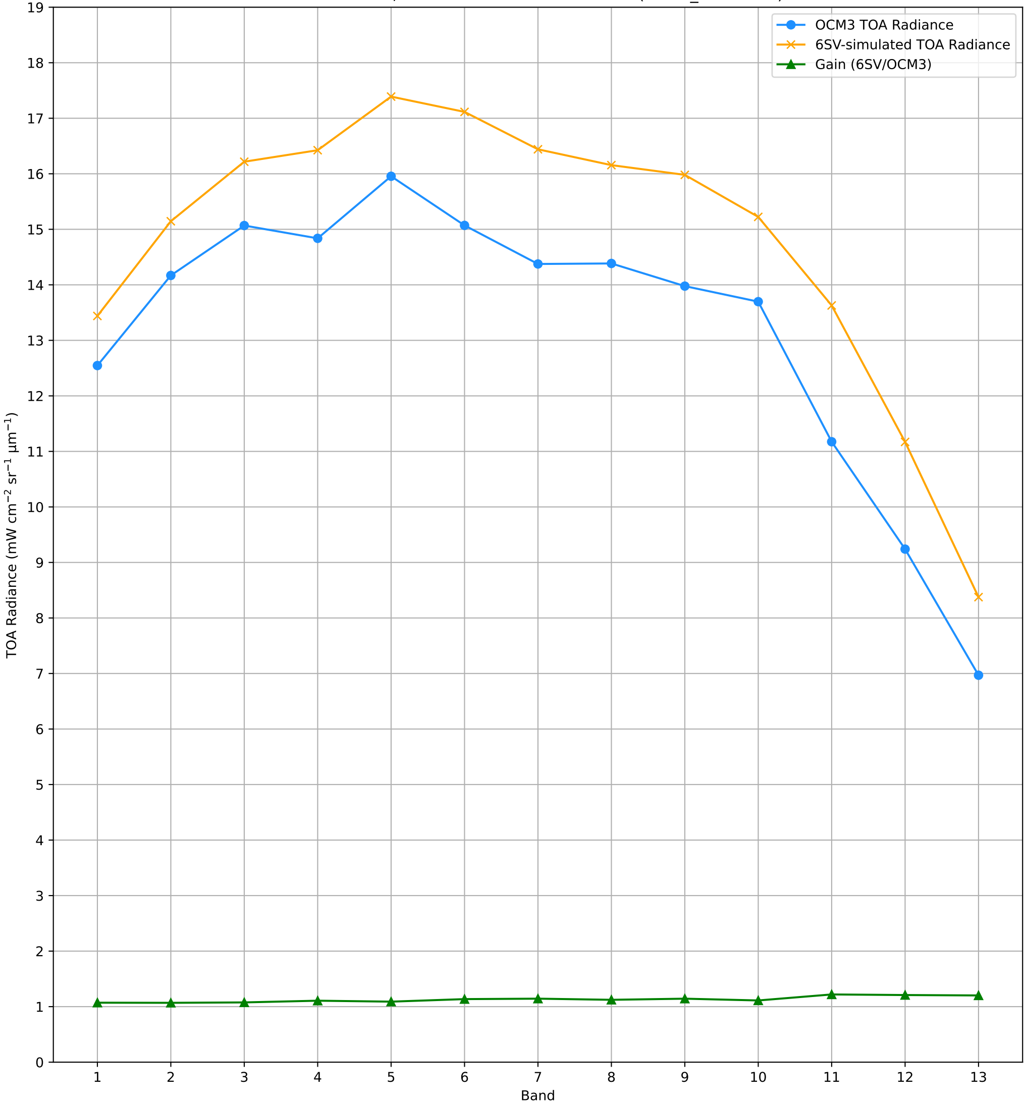
TOA Radiance (OCM3 vs. 6SV) over RVUS RadCalNet Site Lat: 38.497°, Lon: -115.69° - 29-APR-2026 (STRIP_ID: 18086)
