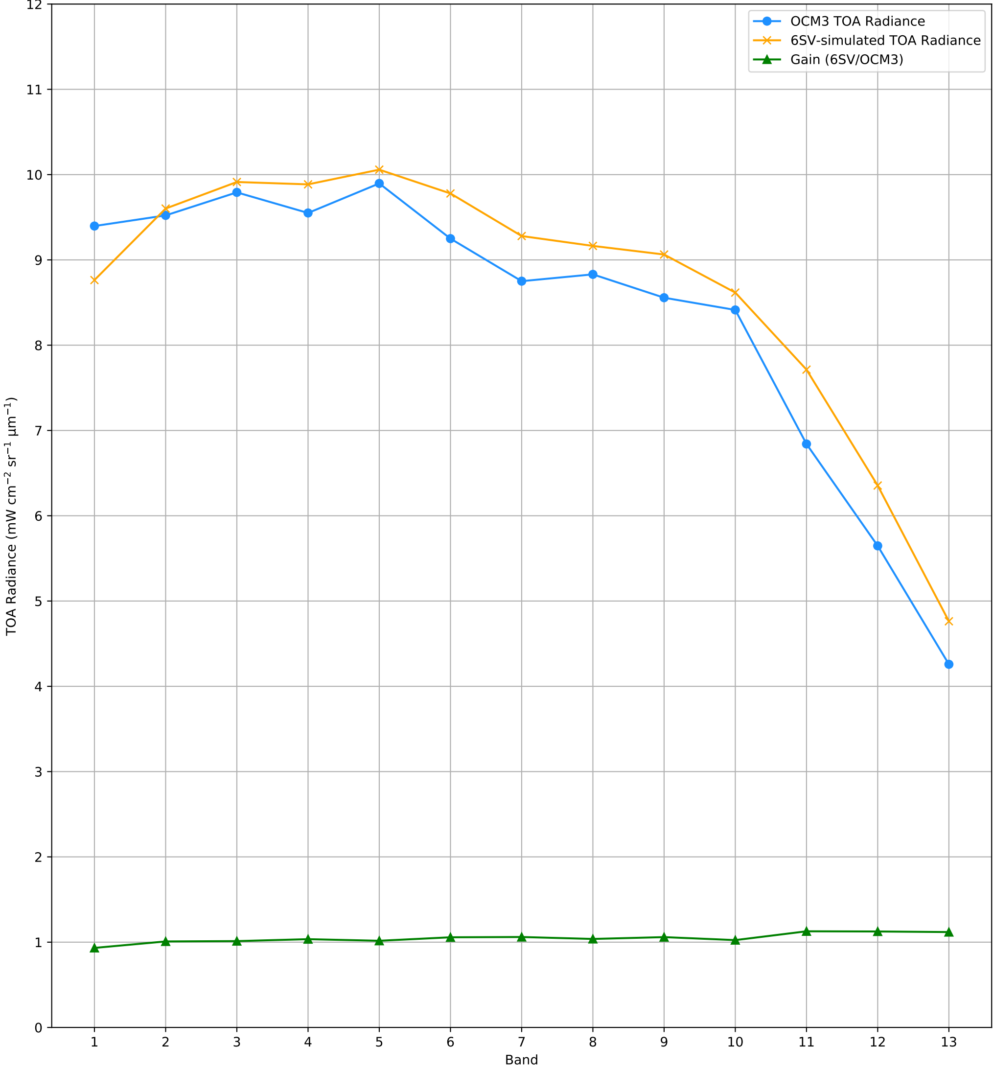
TOA Radiance (OCM3 vs. 6SV) over RVUS RadCalNet Site Lat: 38.497°, Lon: -115.69° - 14-JAN-2025 (STRIP_ID: 11289)
