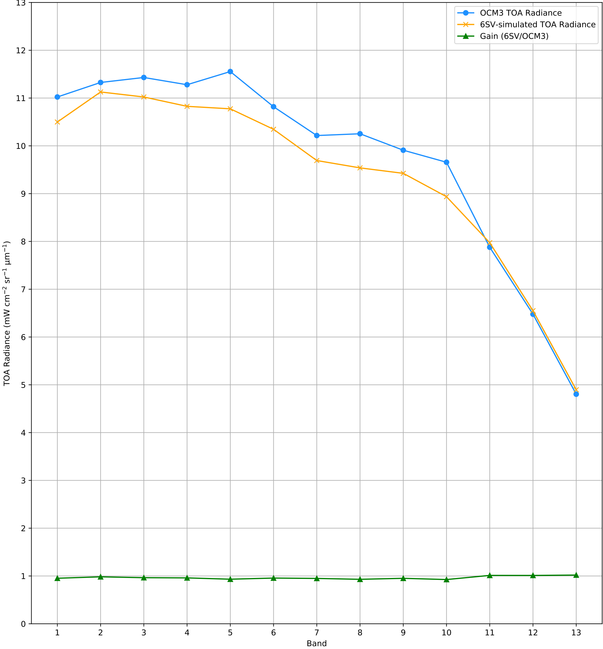
TOA Radiance (OCM3 vs. 6SV) over RVUS RadCalNet Site Lat: 38.497°, Lon: -115.69° - 15-JAN-2025 (STRIP_ID: 11303)
