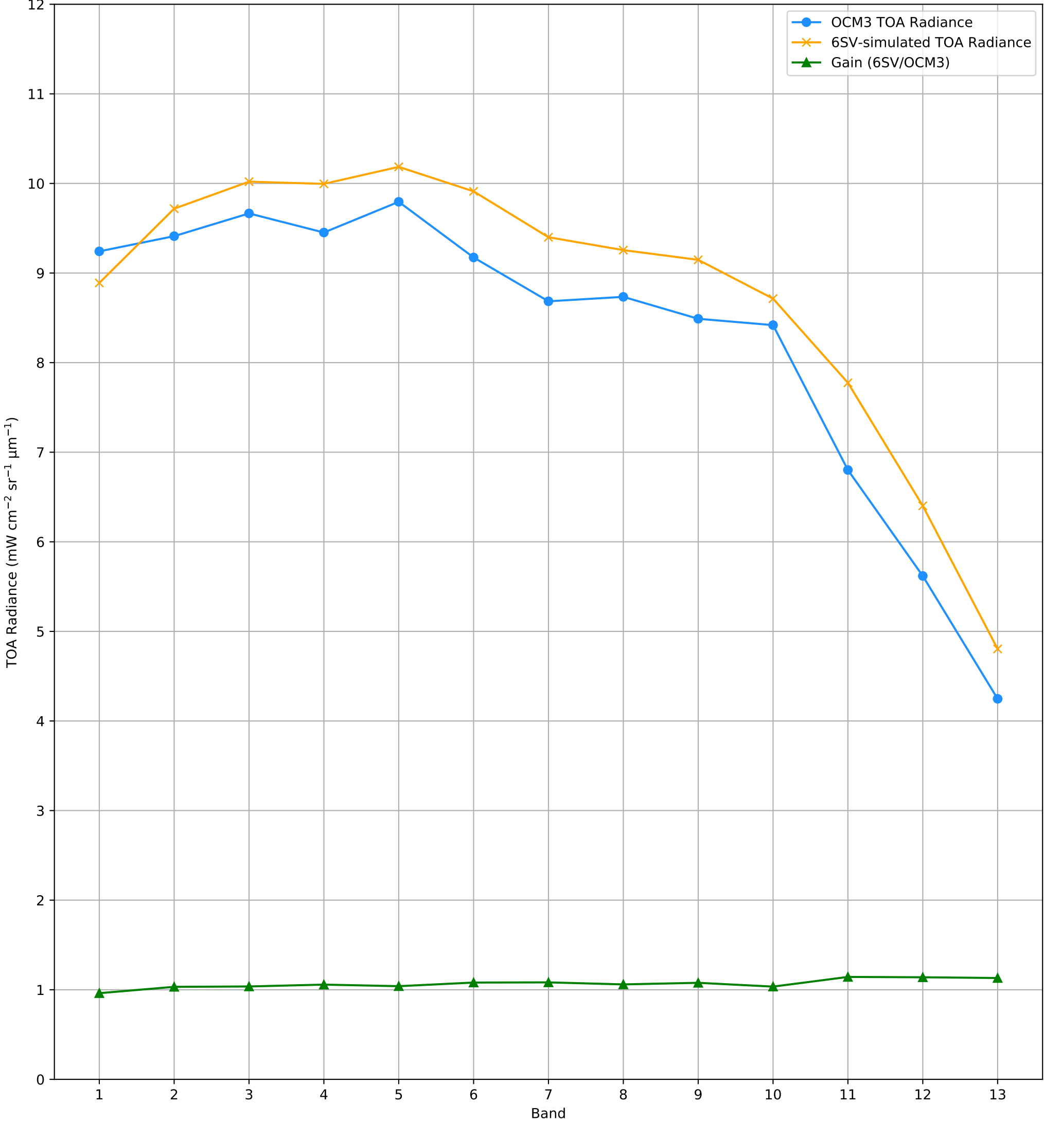
TOA Radiance (OCM3 vs. 6SV) over RVUS RadCalNet Site Lat: 38.497°, Lon: -115.69° - 16-JAN-2025 (STRIP_ID: 11318)
