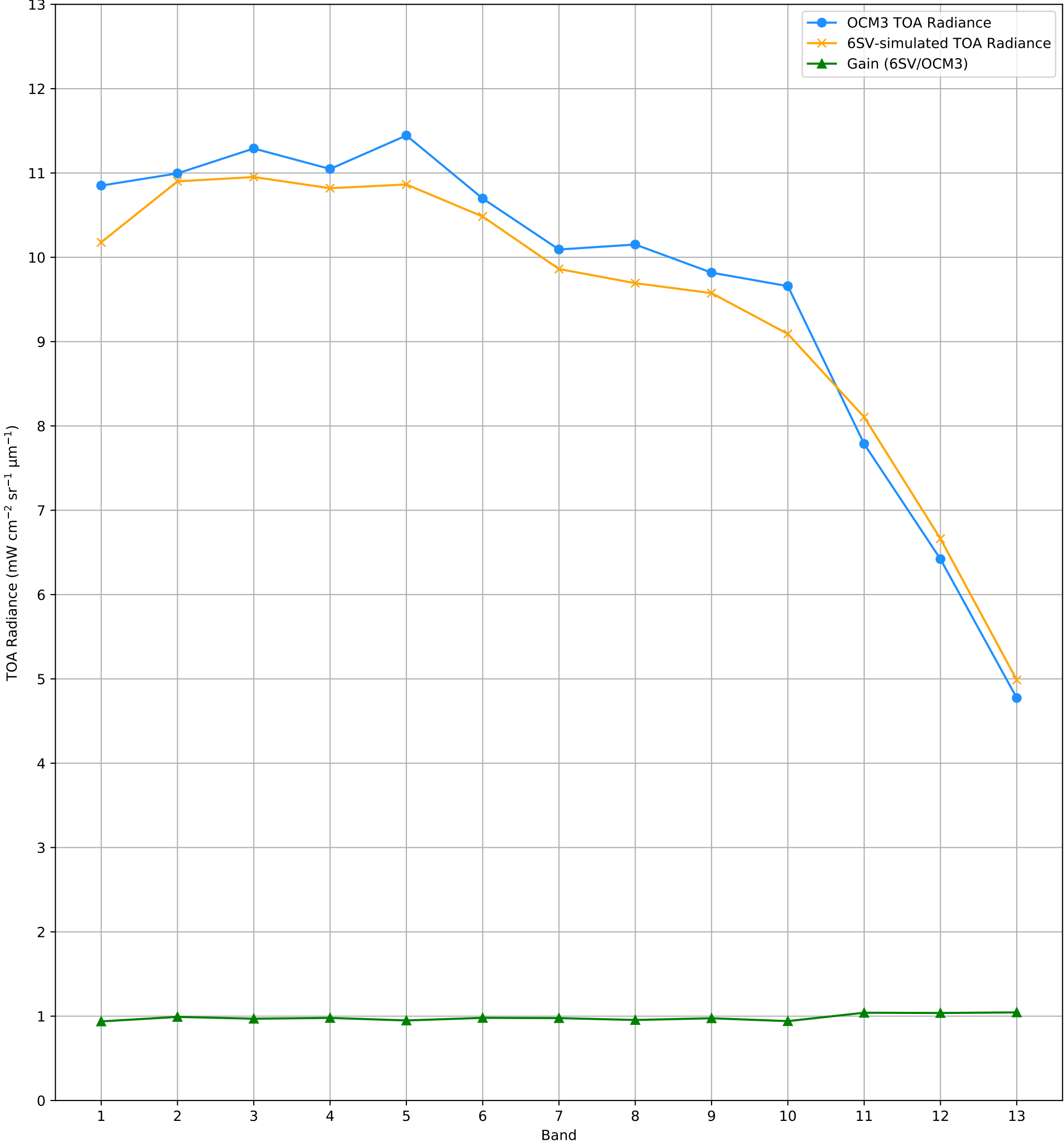
TOA Radiance (OCM3 vs. 6SV) over RVUS RadCalNet Site Lat: 38.497°, Lon: -115.69° - 17-JAN-2025 (STRIP_ID: 11332)
