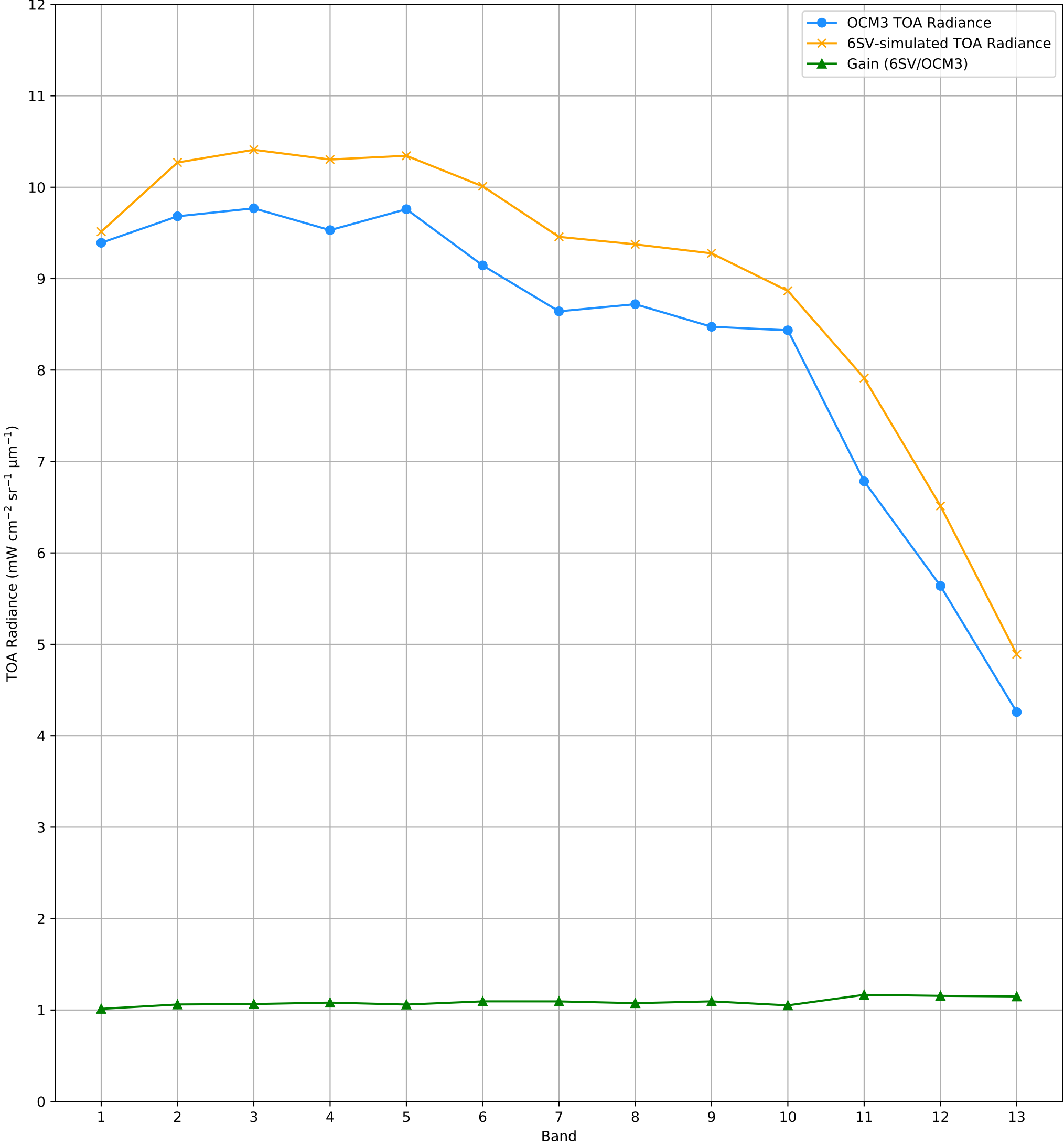
TOA Radiance (OCM3 vs. 6SV) over RVUS RadCalNet Site Lat: 38.497°, Lon: -115.69° - 20-JAN-2025 (STRIP_ID: 11376)
