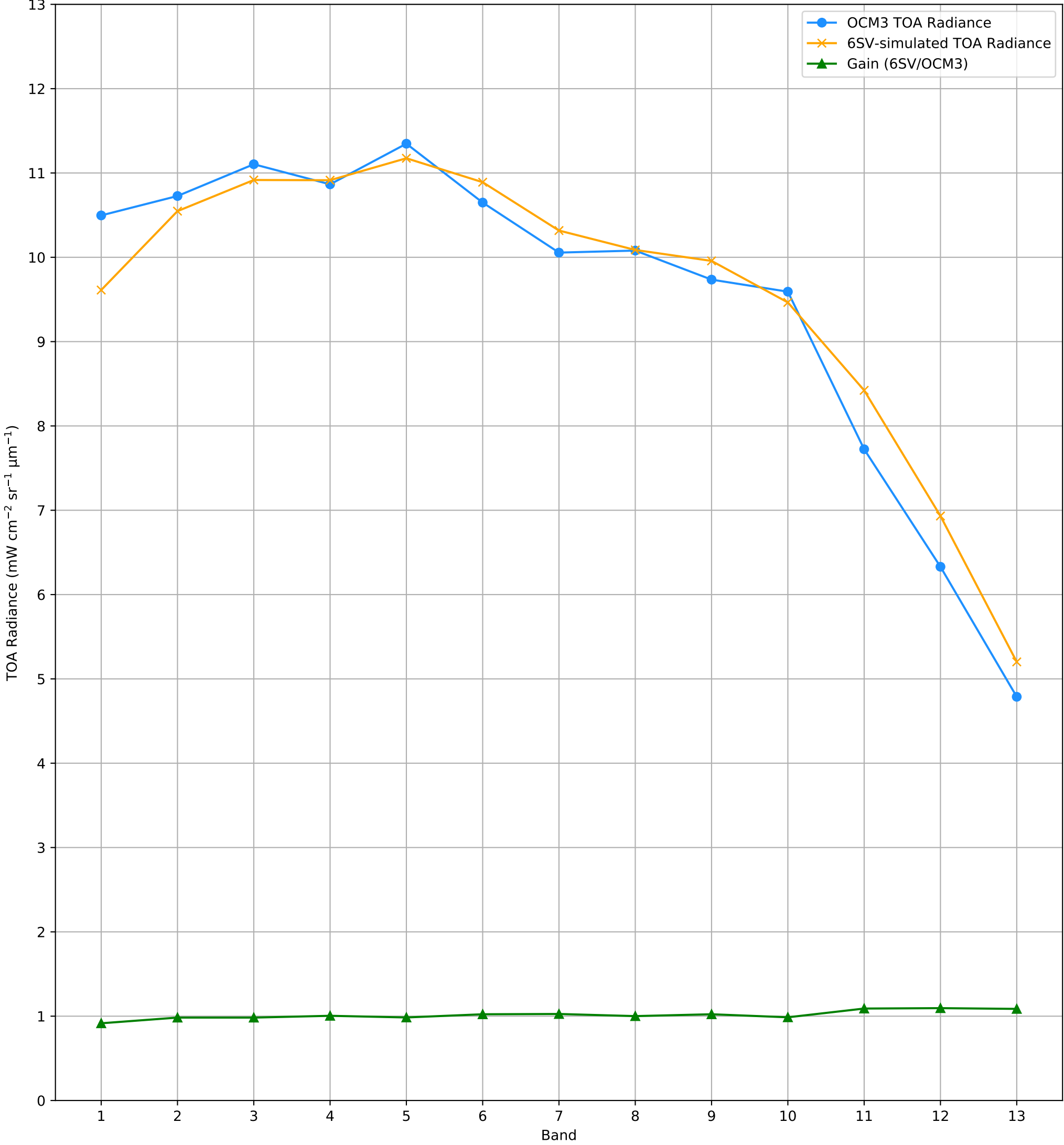
TOA Radiance (OCM3 vs. 6SV) over RVUS RadCalNet Site Lat: 38.497°, Lon: -115.69° - 23-JAN-2025 (STRIP_ID: 11419)
