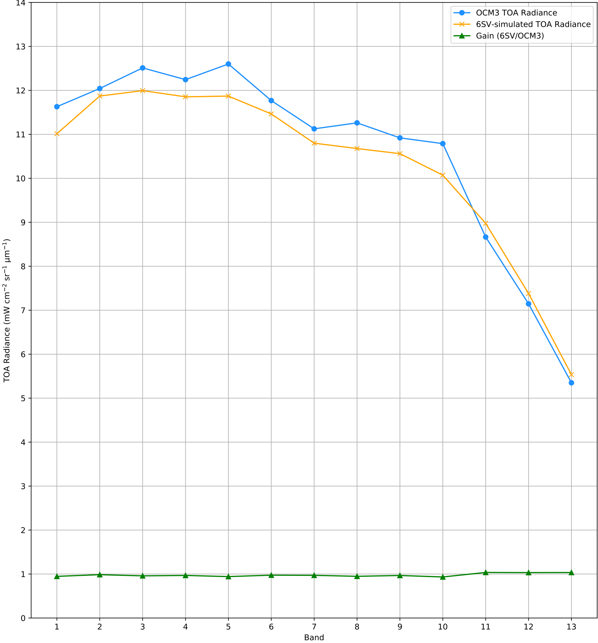
TOA Radiance (OCM3 vs. 6SV) over RVUS RadCalNet Site Lat: 38.497°, Lon: -115.69° - 30-JAN-2025 (STRIP_ID: 11520)
