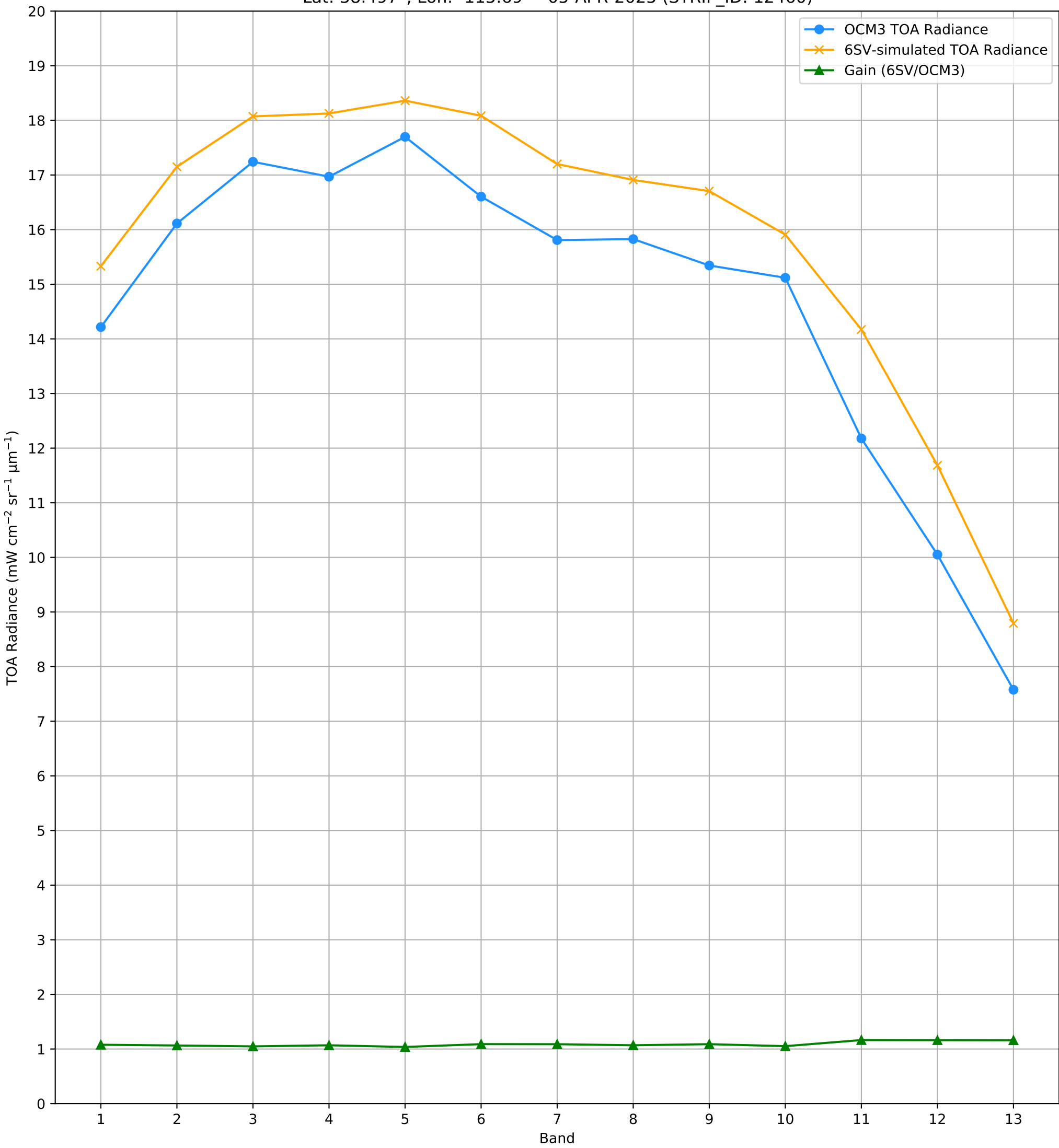
TOA Radiance (OCM3 vs. 6SV) over RVUS RadCalNet Site Lat: 38.497°, Lon: -115.69° - 05-APR-2025 (STRIP_ID: 12460)
