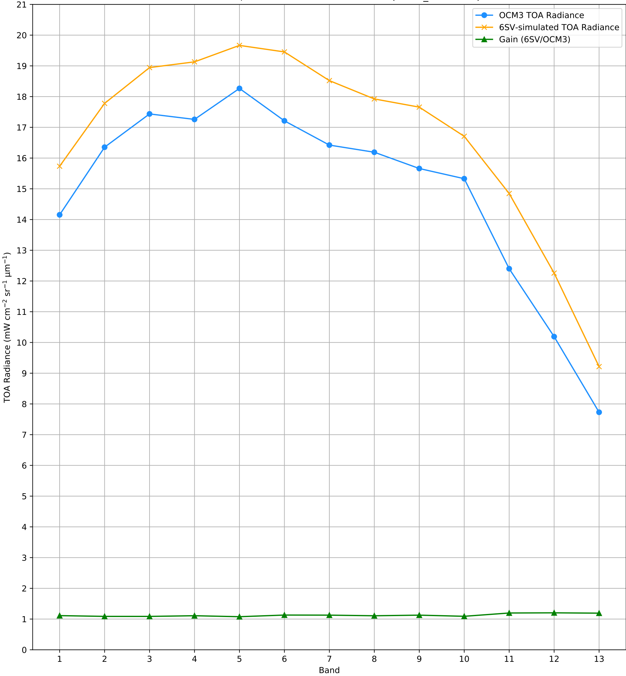
TOA Radiance (OCM3 vs. 6SV) over RVUS RadCalNet Site Lat: 38.497°, Lon: -115.69° - 09-APR-2025 (STRIP_ID:12518)
