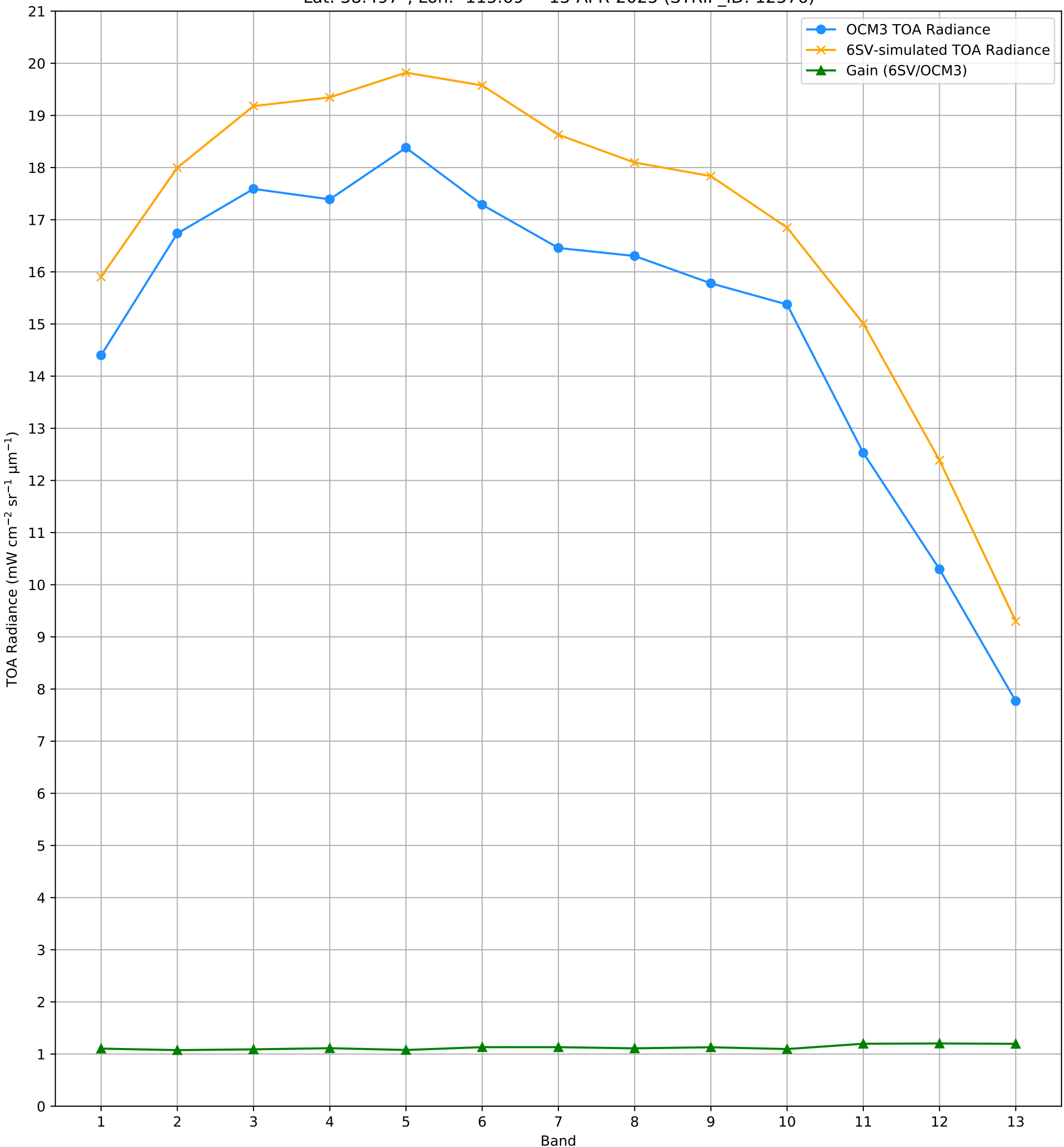
TOA Radiance (OCM3 vs. 6SV) over RVUS RadCalNet Site Lat: 38.497°, Lon: -115.69° - 13-APR-2025 (STRIP_ID: 12576)
