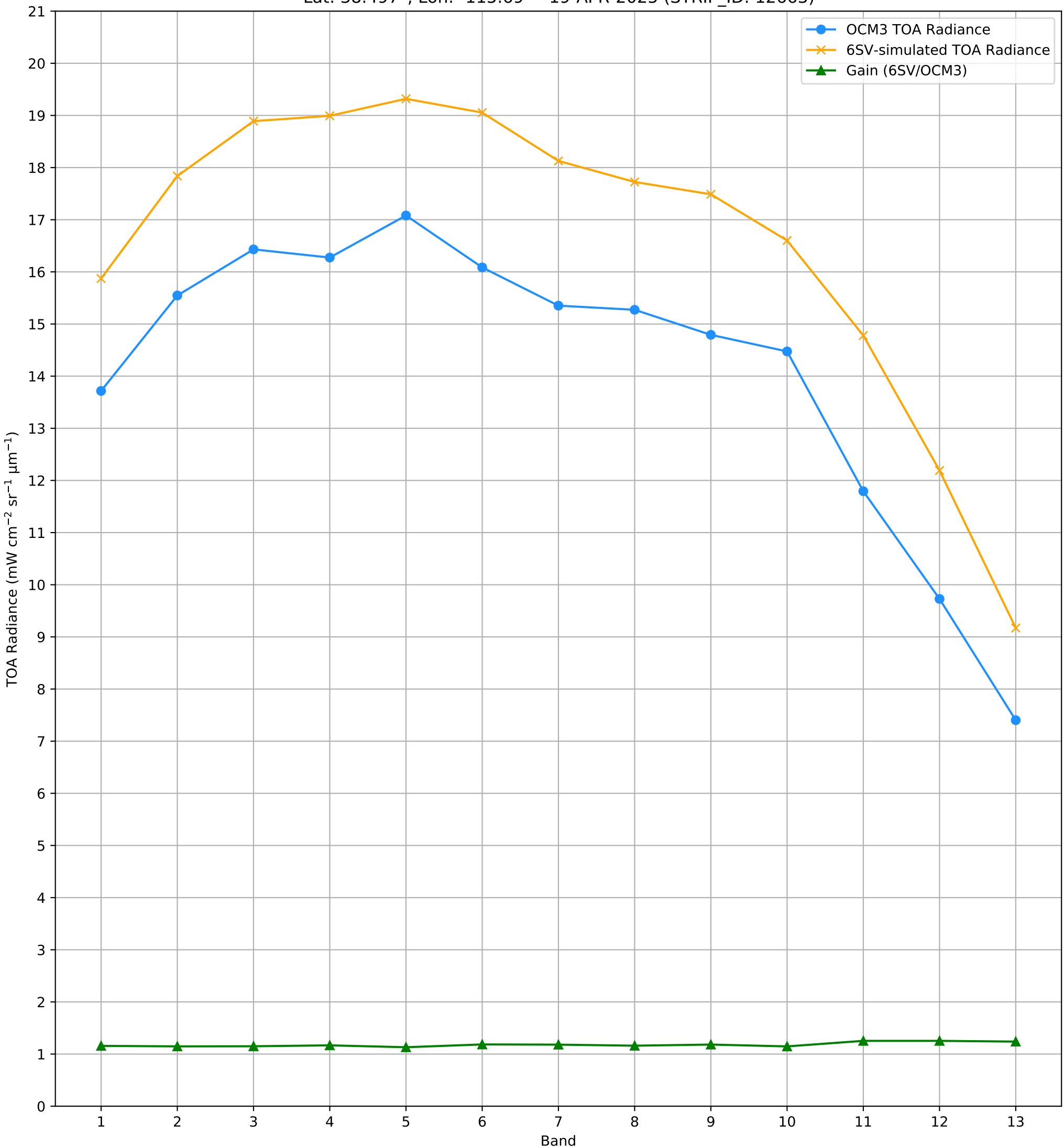
TOA Radiance (OCM3 vs. 6SV) over RVUS RadCalNet Site Lat: 38.497°, Lon: -115.69° - 19-APR-2025 (STRIP_ID: 12663)
