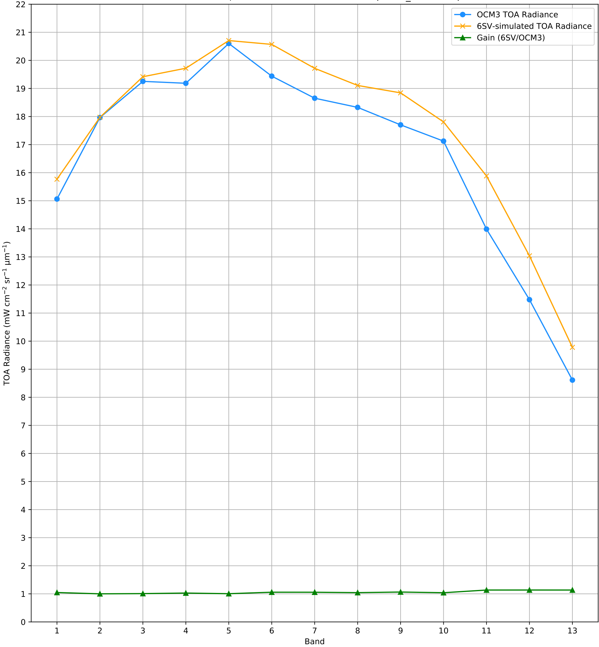
TOA Radiance (OCM3 vs. 6SV) over RVUS RadCalNet Site Lat: 38.497°, Lon: -115.69° - 09-MAY-2025 (STRIP_ID: 12952)
