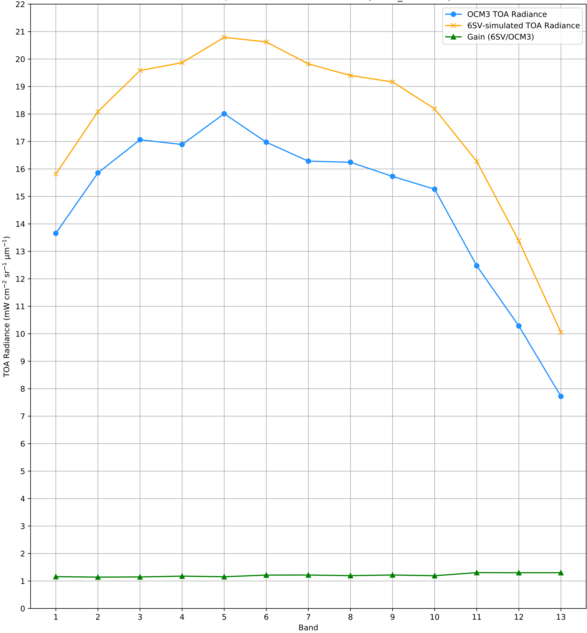
TOA Radiance (OCM3 vs. 6SV) over RVUS RadCalNet Site Lat: 38.497°, Lon: -115.69° - 29-MAY-2025 (STRIP_ID: 13241)
