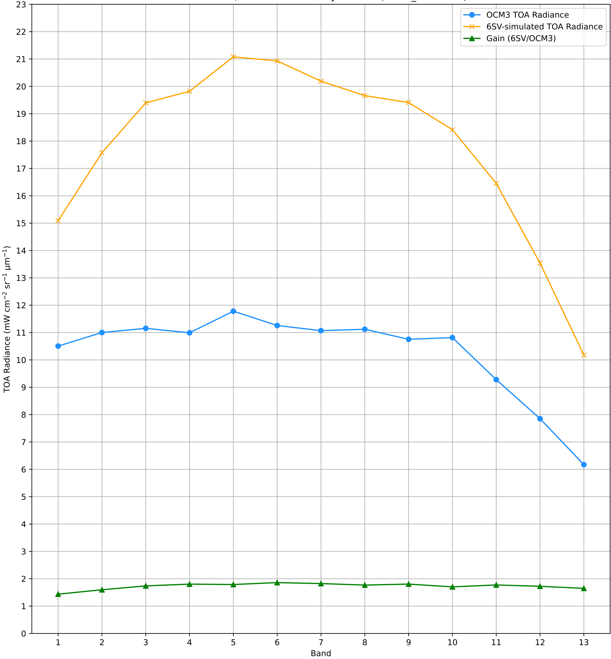
TOA Radiance (OCM3 vs. 6SV) over RVUS RadCalNet Site Lat: 38.497°, Lon: -115.69° - 28-JUN-2025 (STRIP_ID: 13675)
