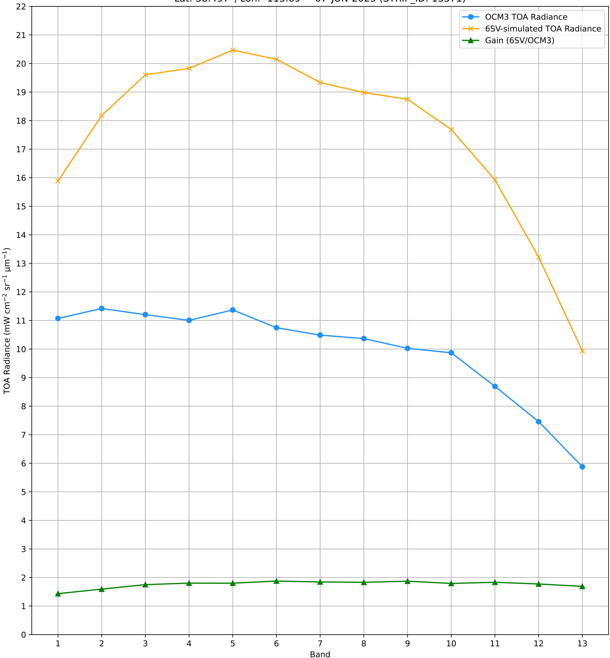
TOA Radiance (OCM3 vs. 6SV) over RVUS RadCalNet Site Lat: 38.497°, Lon: -115.69° - 07-JUN-2025 (STRIP_ID: 13371)
