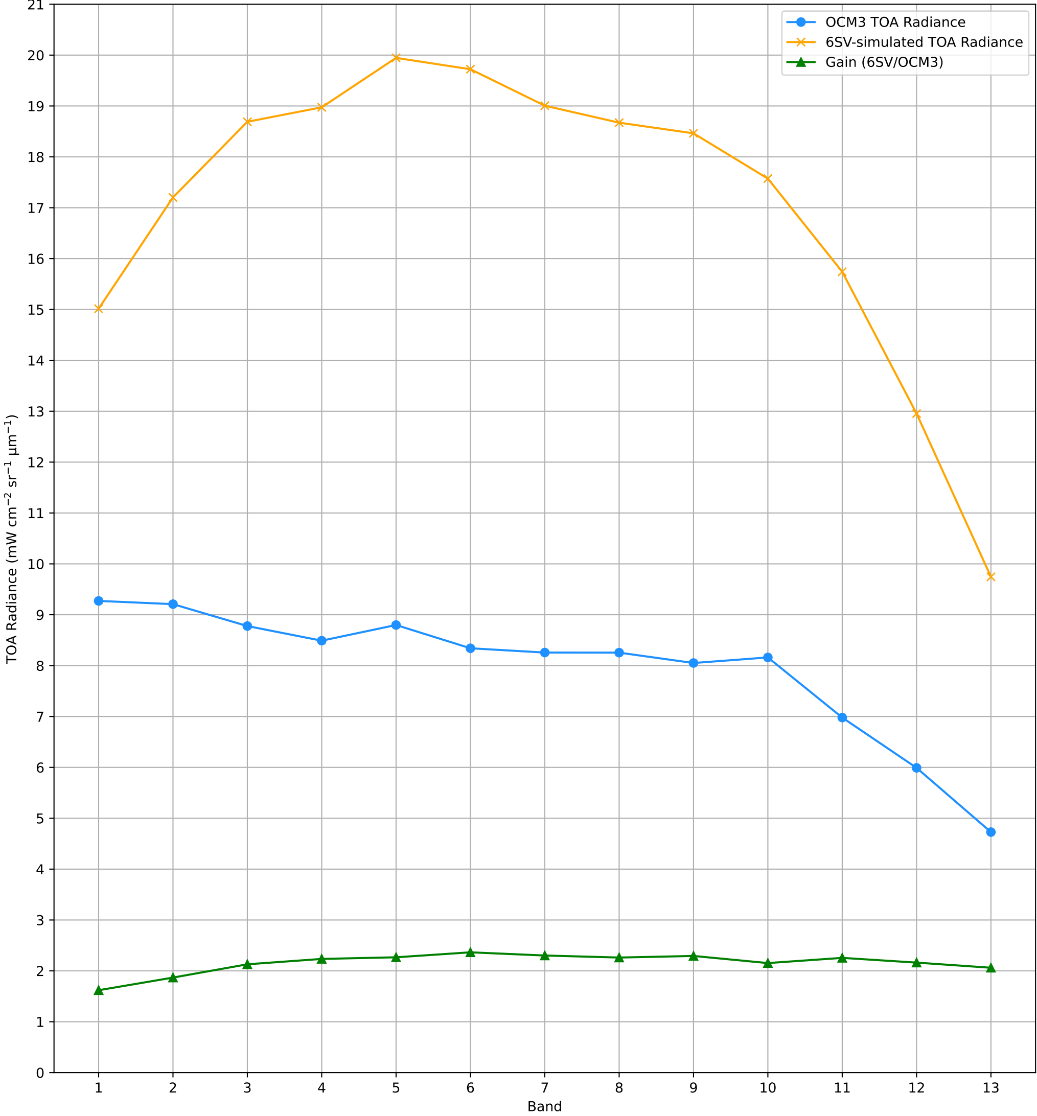
TOA Radiance (OCM3 vs. 6SV) over RVUS RadCalNet Site Lat: 38.497°, Lon: -115.69° - 12-JUN-2025 (STRIP_ID: 13444)
