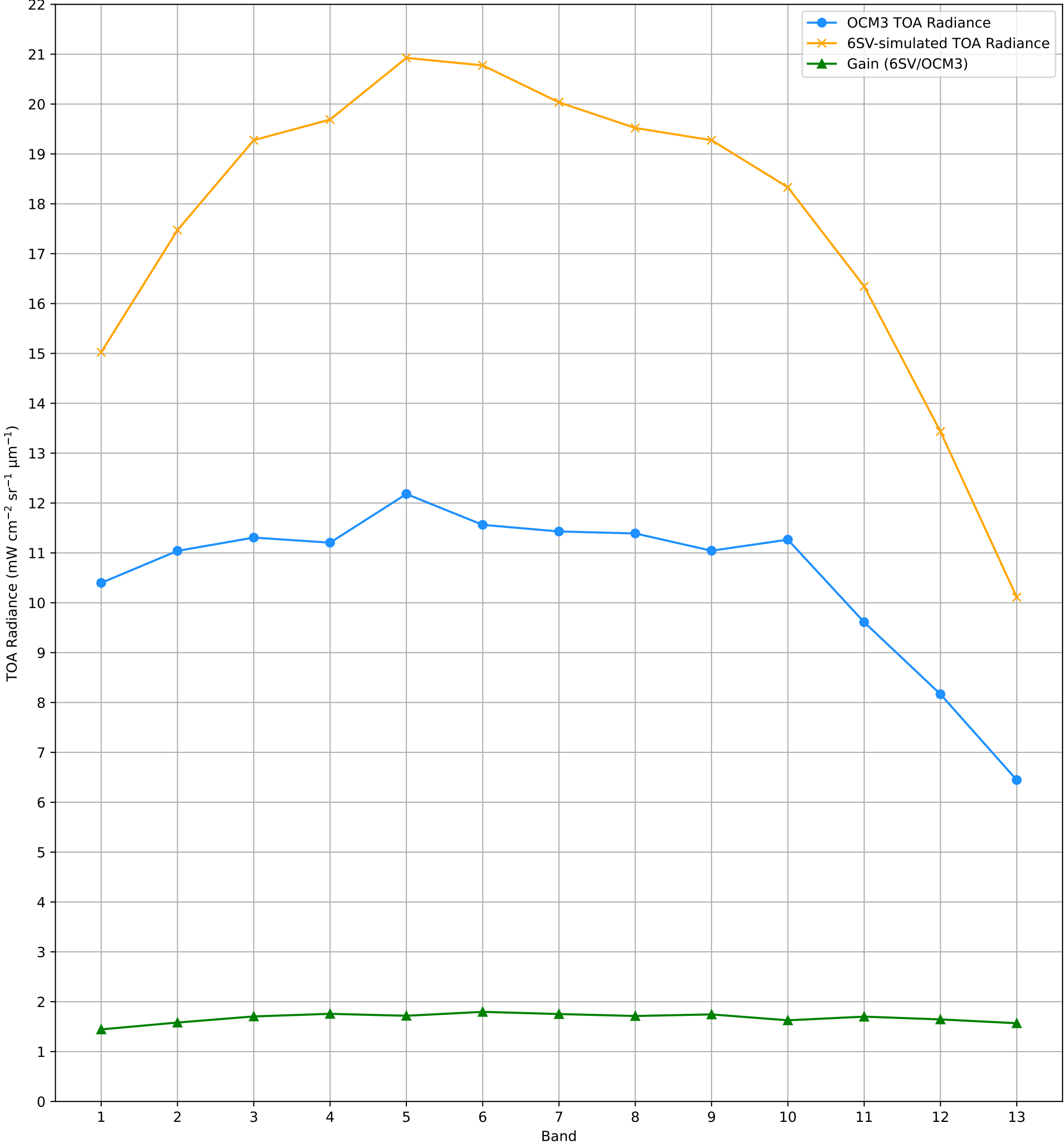
TOA Radiance (OCM3 vs. 6SV) over RVUS RadCalNet Site Lat: 38.497°, Lon: -115.69° - 13-JUN-2025 (STRIP_ID: 13458)
