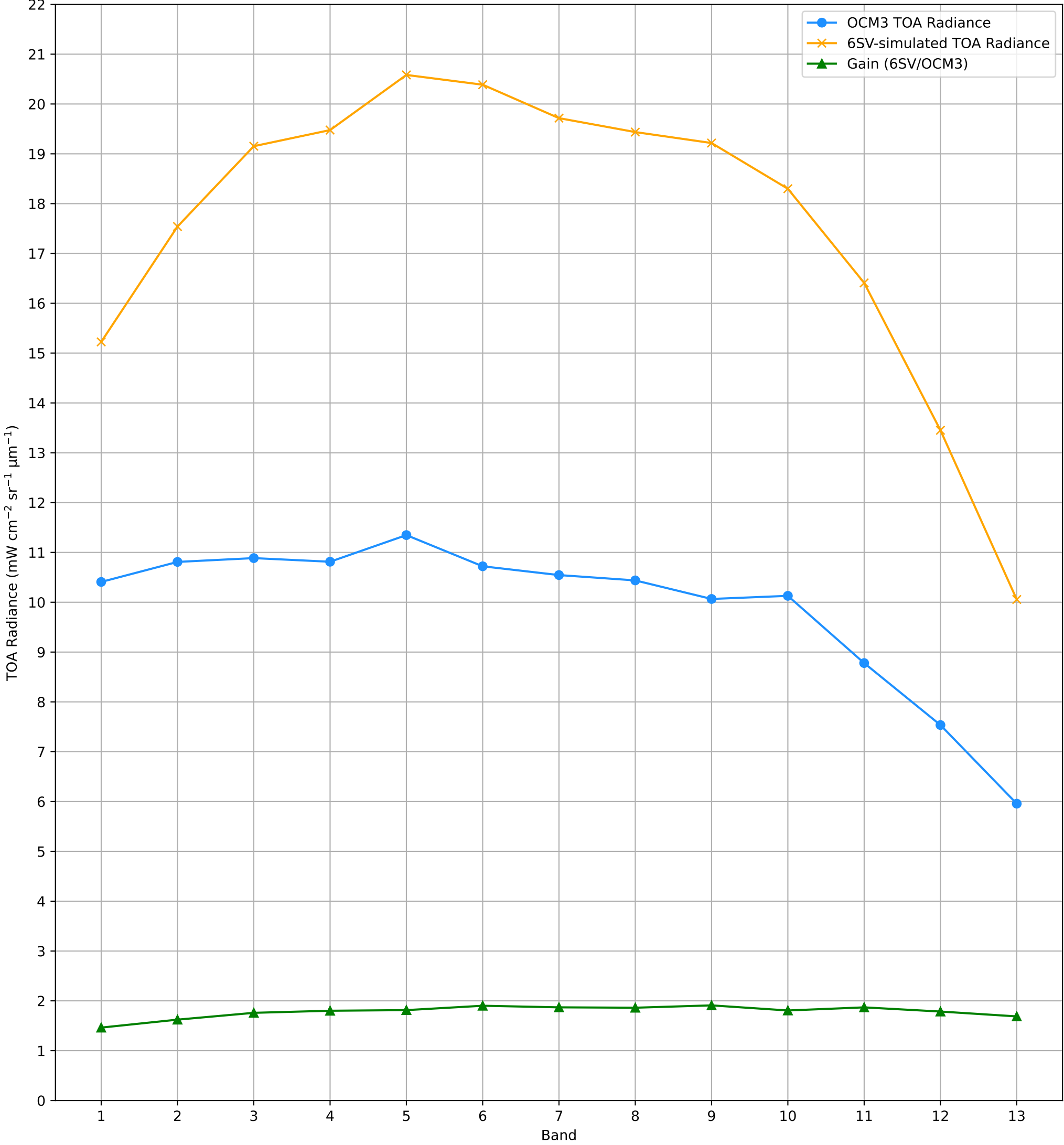
TOA Radiance (OCM3 vs. 6SV) over RVUS RadCalNet Site Lat: 38.497°, Lon: -115.69° - 20-JUN-2025 (STRIP_ID: 13559)
