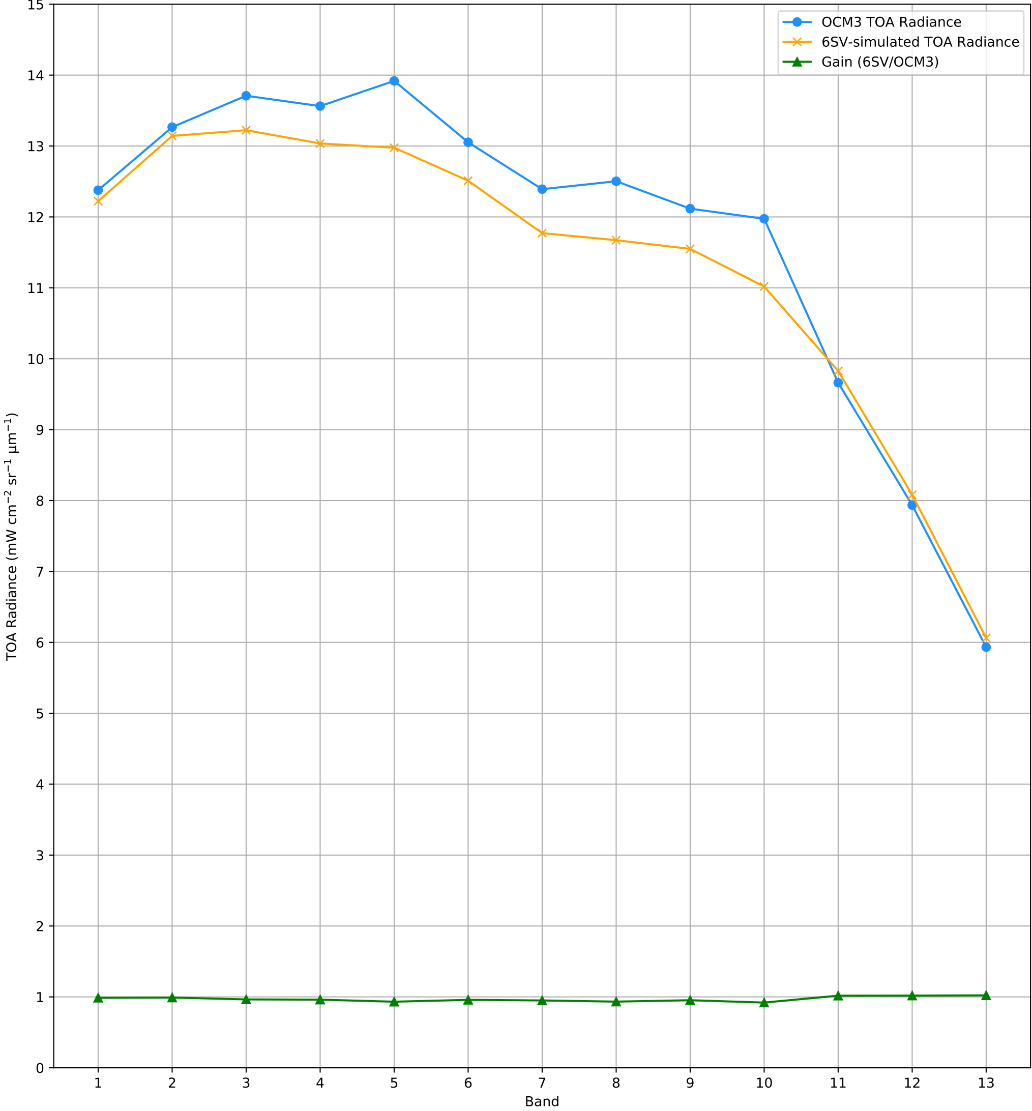
TOA Radiance (OCM3 vs. 6SV) over RVUS RadCalNet Site Lat: 38.497°, Lon: -115.69° - 10-FEB-2025 (STRIP_ID: 11679)
