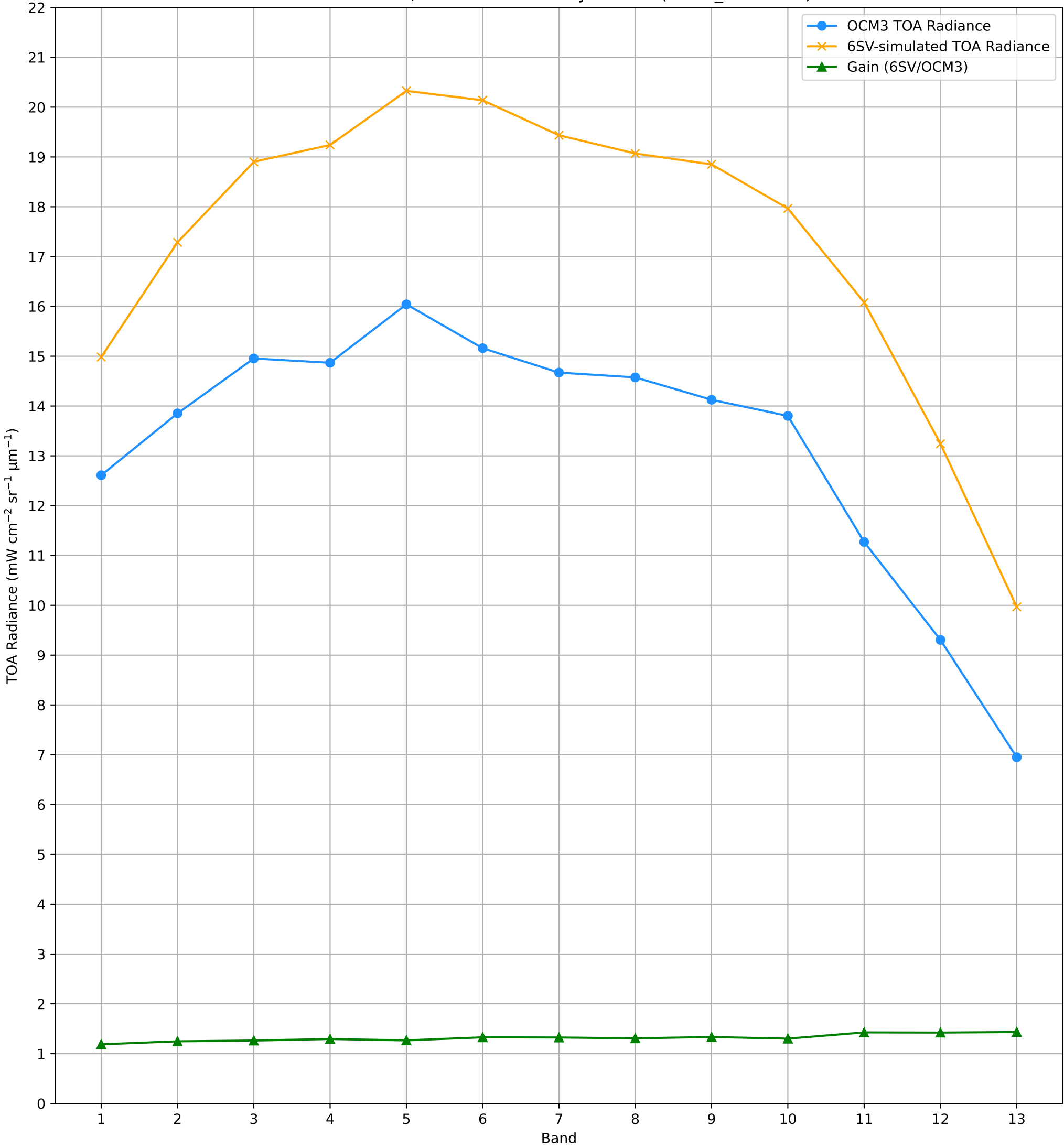
TOA Radiance (OCM3 vs. 6SV) over RVUS RadCalNet Site Lat: 38.497°, Lon: -115.69° - 05-JUL-2025 (STRIP_ID: 13776)
