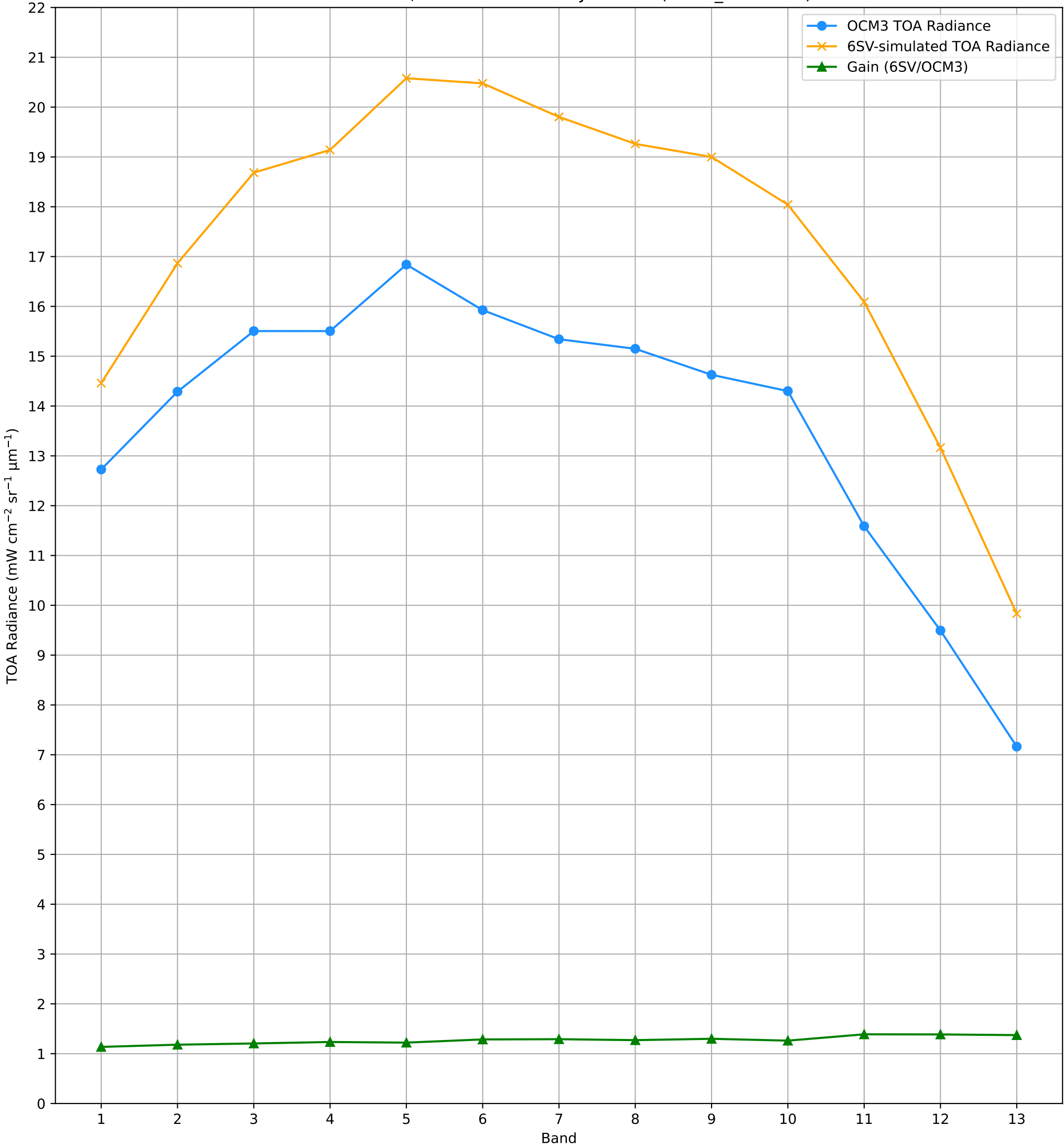
TOA Radiance (OCM3 vs. 6SV) over RVUS RadCalNet Site Lat: 38.497°, Lon: -115.69° - 09-JUL-2025 (STRIP_ID: 13834)
