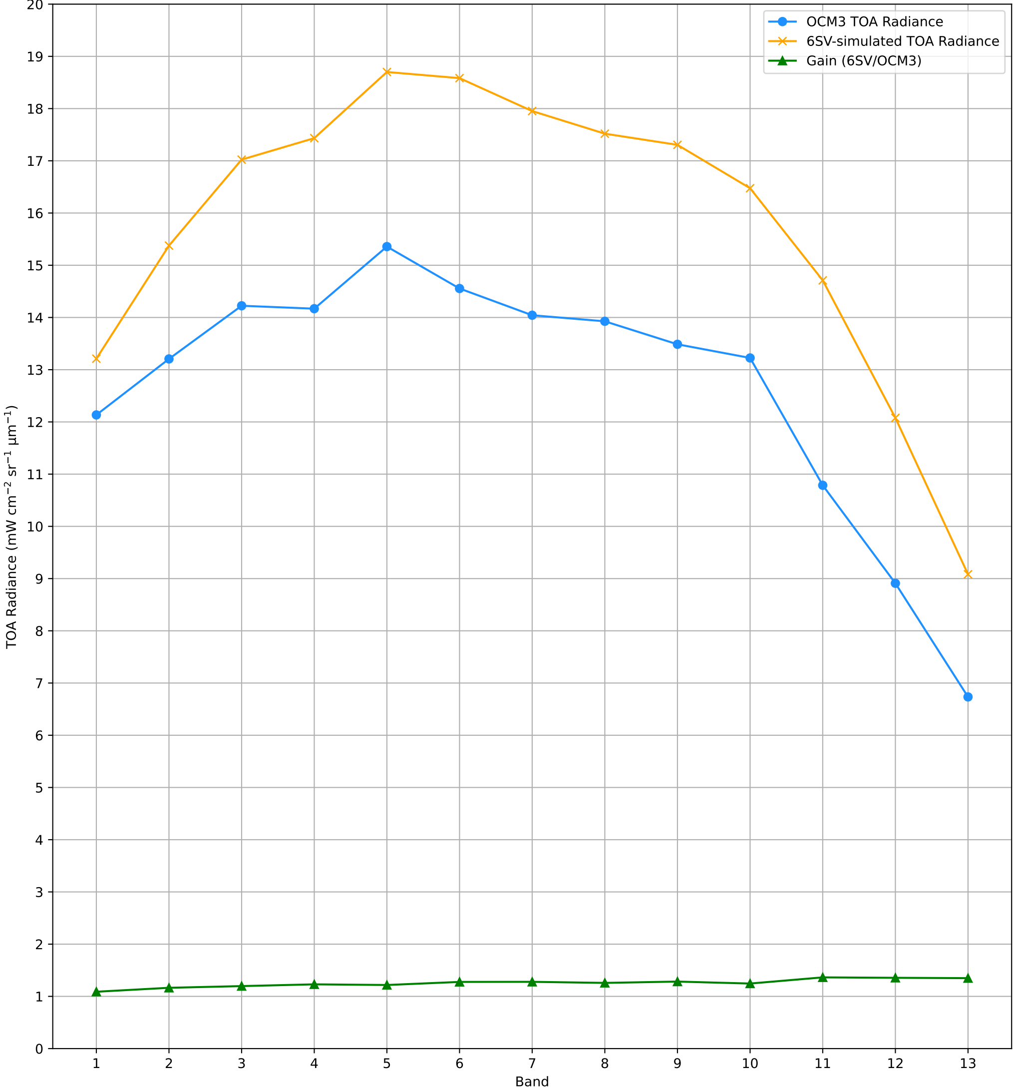
TOA Radiance (OCM3 vs. 6SV) over RVUS RadCalNet Site Lat: 38.497°, Lon: -115.69° - 28-JUL-2025 (STRIP_ID: 14109)
