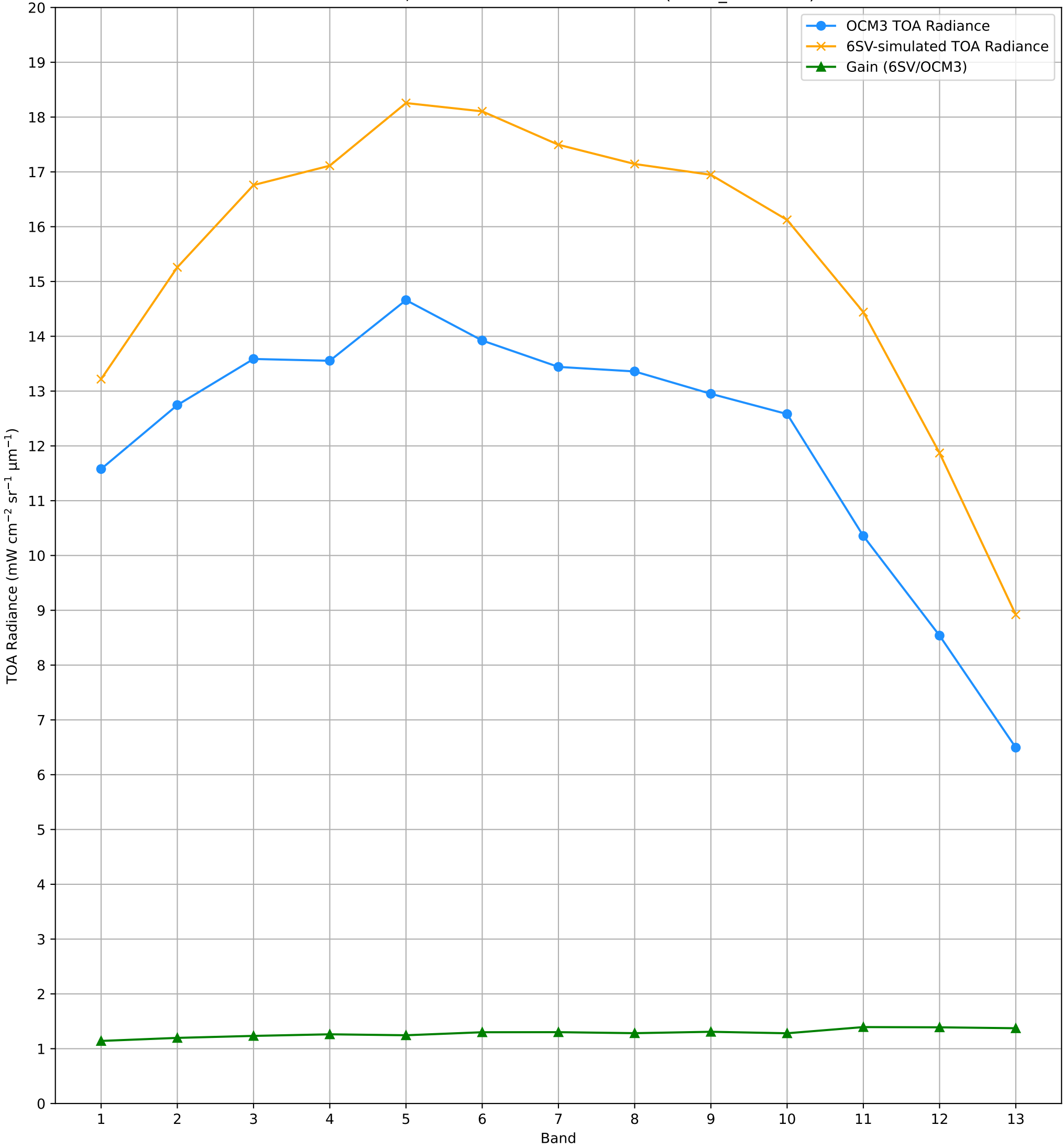
TOA Radiance (OCM3 vs. 6SV) over RVUS RadCalNet Site Lat: 38.497°, Lon: -115.69° - 01-AUG-2025 (STRIP_ID: 14167)
