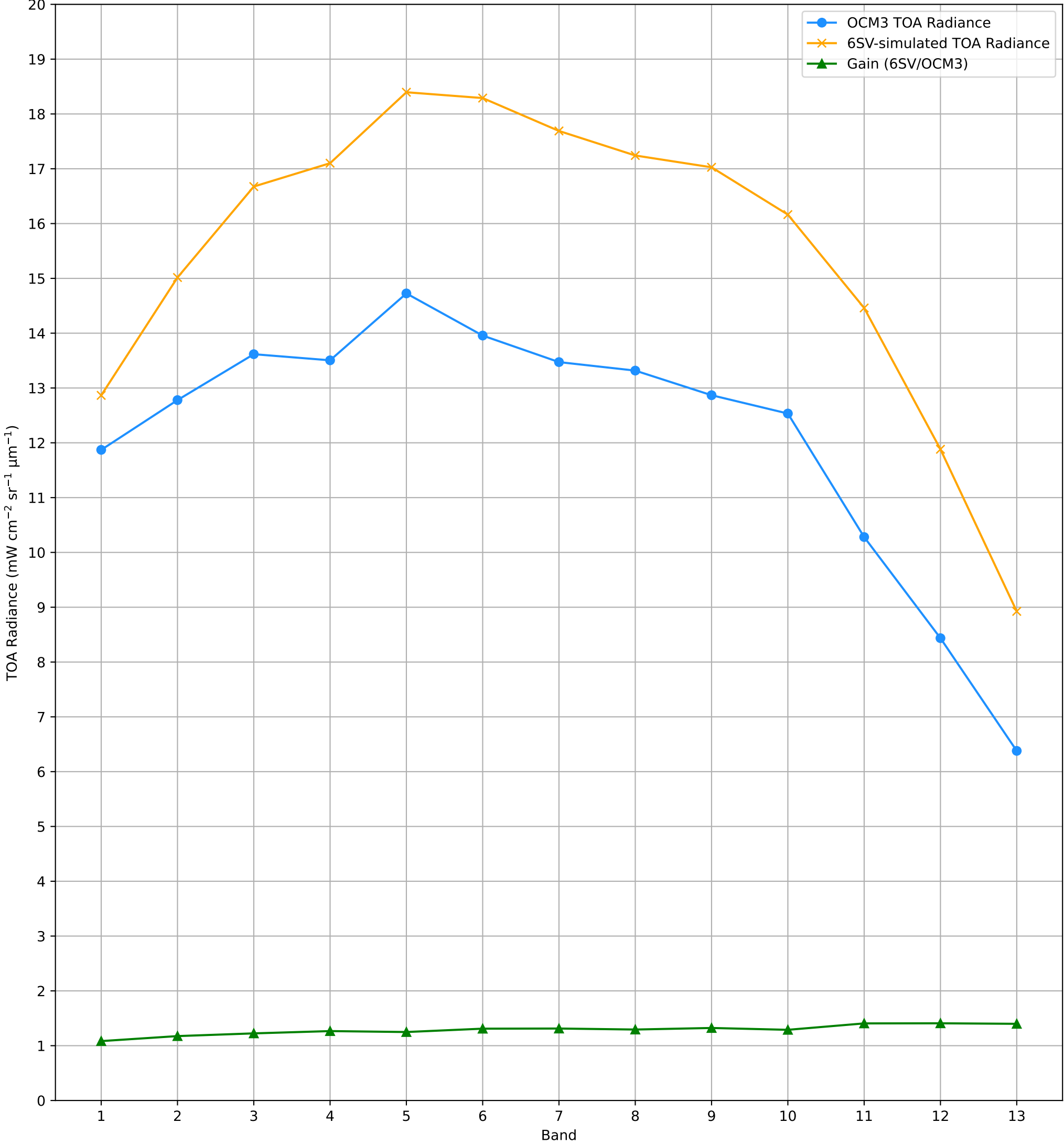
TOA Radiance (OCM3 vs. 6SV) over RVUS RadCalNet Site Lat: 38.497°, Lon: -115.69° - 08-AUG-2025 (STRIP_ID: 14268)
