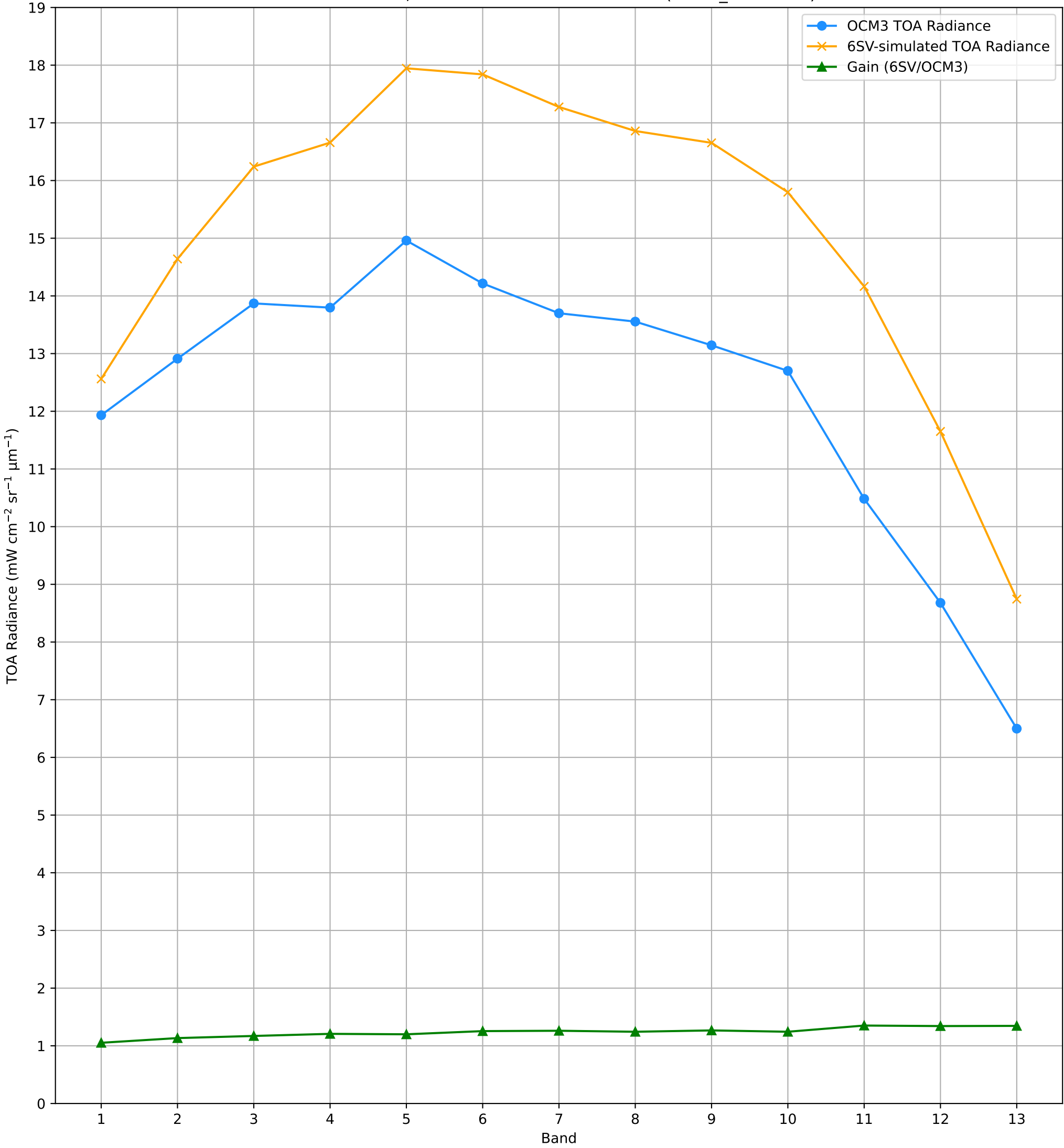
TOA Radiance (OCM3 vs. 6SV) over RVUS RadCalNet Site Lat: 38.497°, Lon: -115.69° - 10-AUG-2025 (STRIP_ID: 14297)
