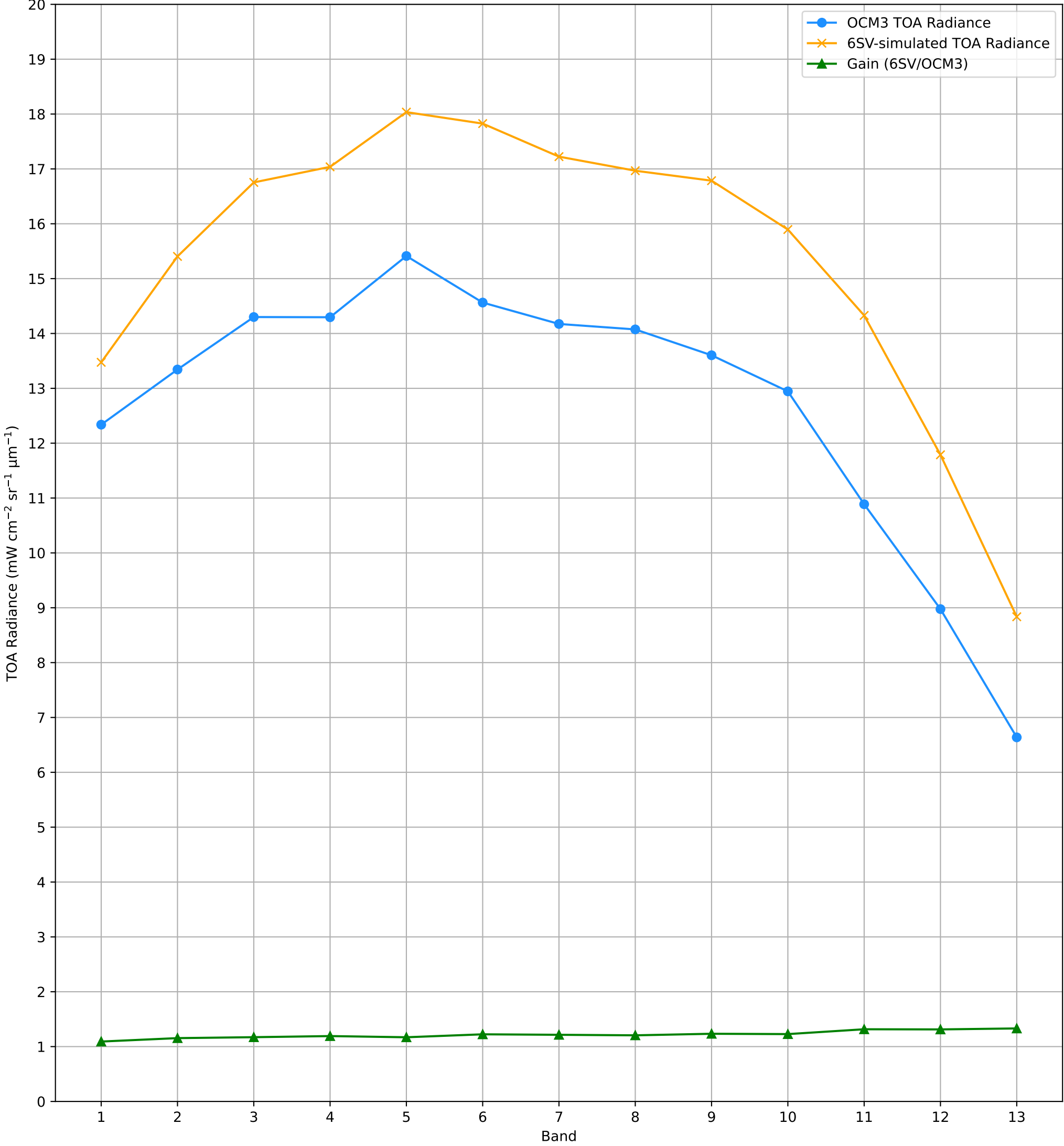
TOA Radiance (OCM3 vs. 6SV) over RVUS RadCalNet Site Lat: 38.497°, Lon: -115.69° - 11-AUG-2025 (STRIP_ID: 14311)
