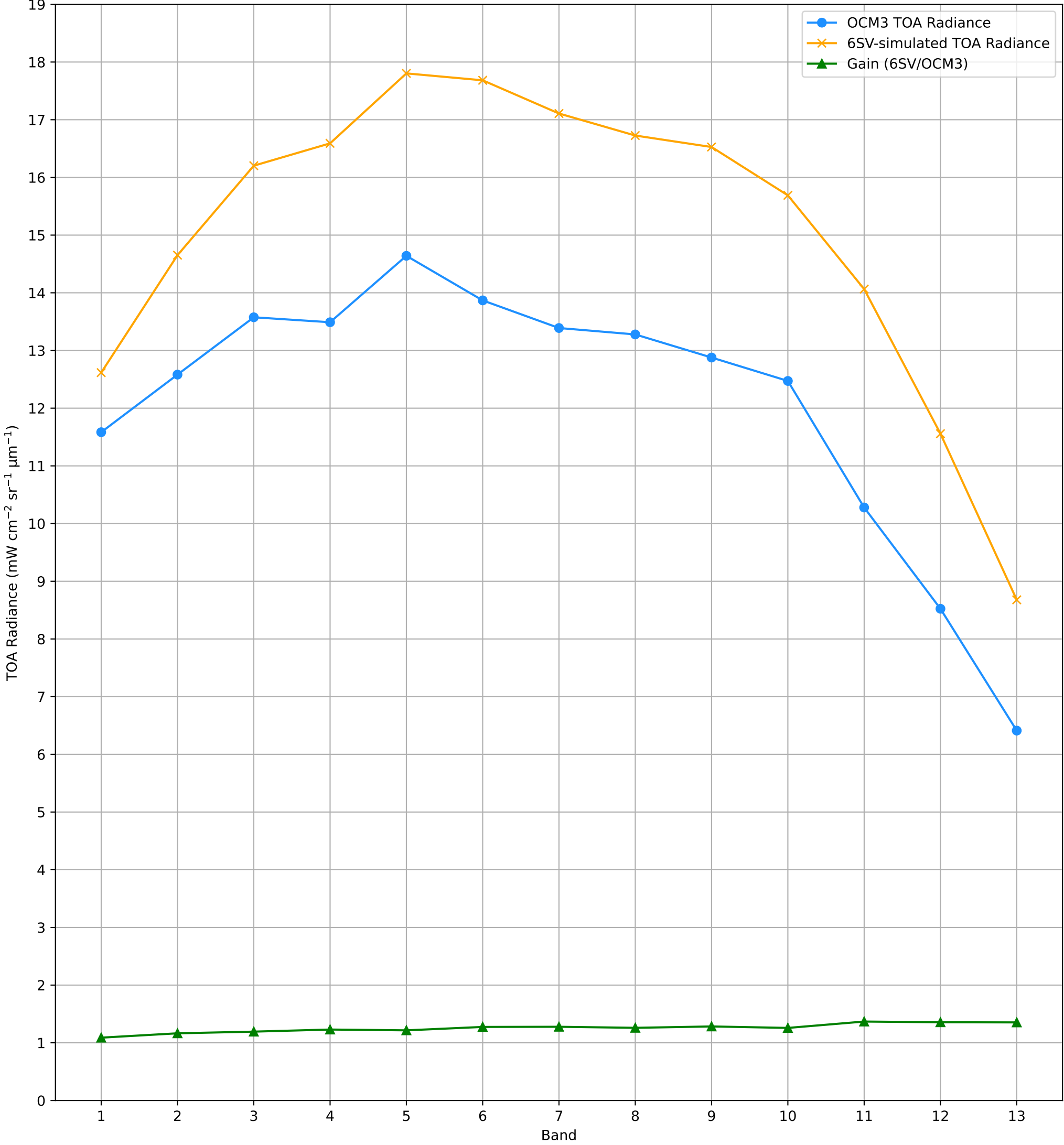
TOA Radiance (OCM3 vs. 6SV) over RVUS RadCalNet Site Lat: 38.497°, Lon: -115.69° - 12-AUG-2025 (STRIP_ID: 14326)
