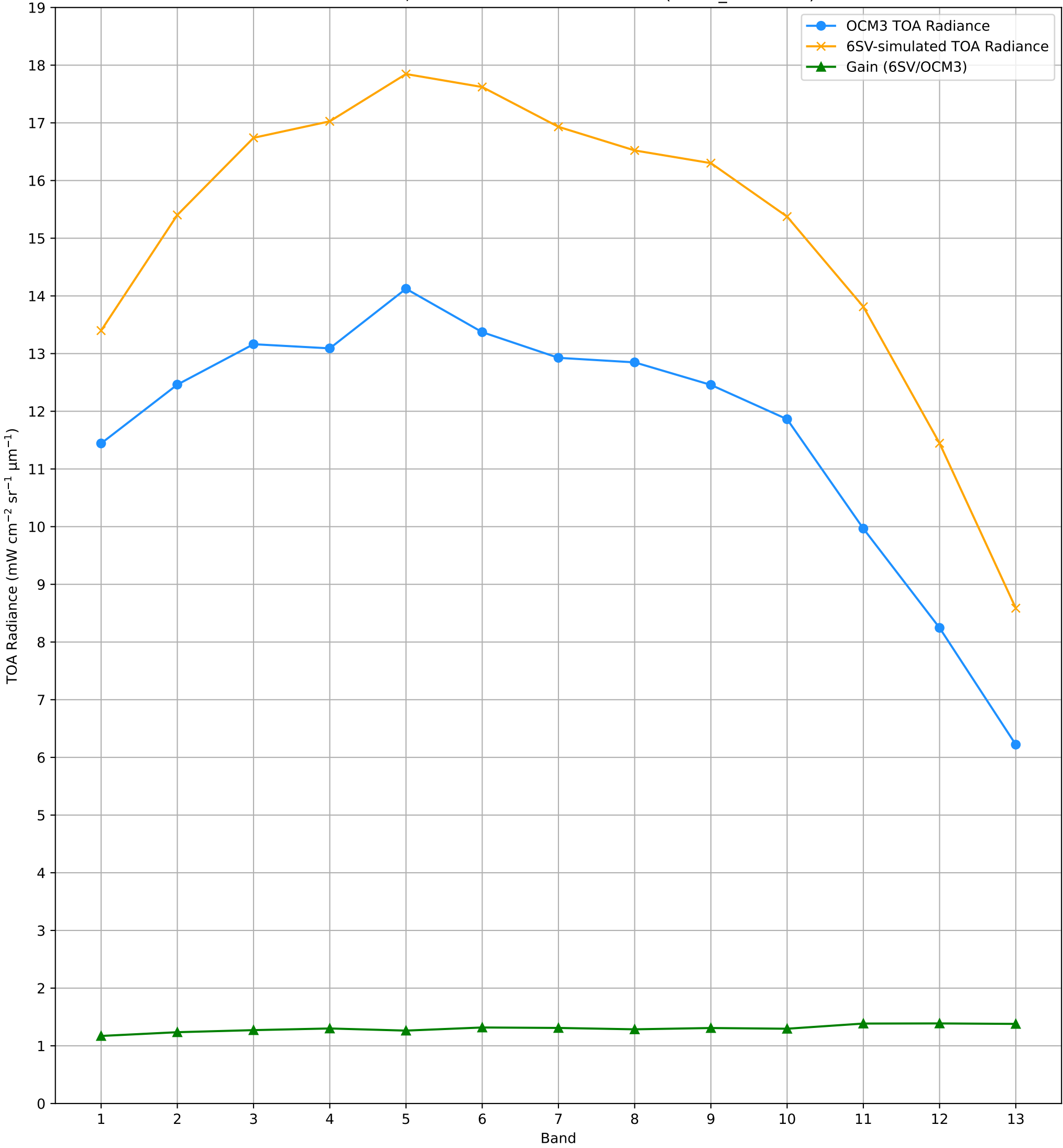
TOA Radiance (OCM3 vs. 6SV) over RVUS RadCalNet Site Lat: 38.497°, Lon: -115.69° - 14-AUG-2025 (STRIP_ID: 14355)
