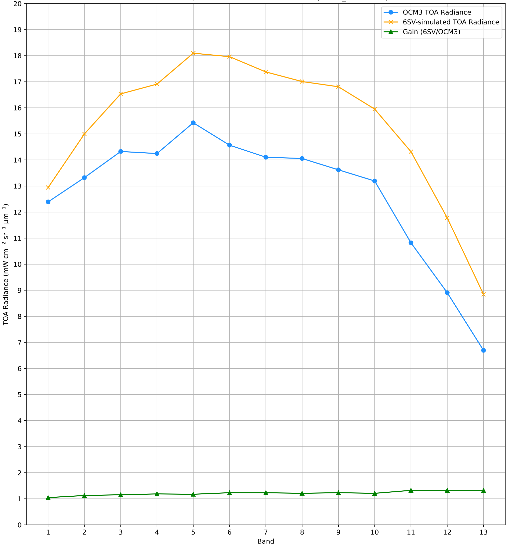
TOA Radiance (OCM3 vs. 6SV) over RVUS RadCalNet Site Lat: 38.497°, Lon: -115.69° - 15-AUG-2025 (STRIP_ID: 14369)
