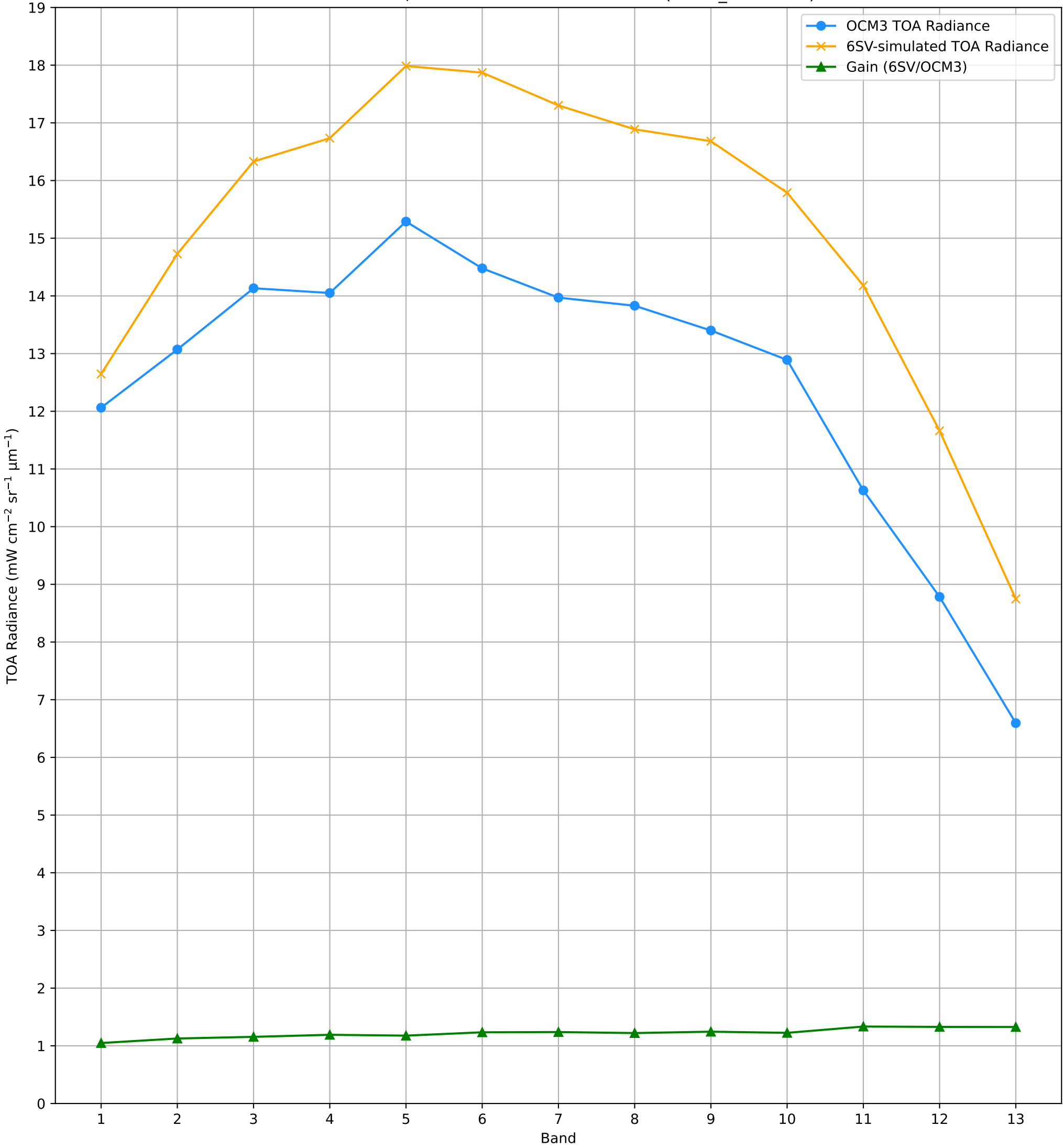
TOA Radiance (OCM3 vs. 6SV) over RVUS RadCalNet Site Lat: 38.497°, Lon: -115.69° - 17-AUG-2025 (STRIP_ID: 14398)
