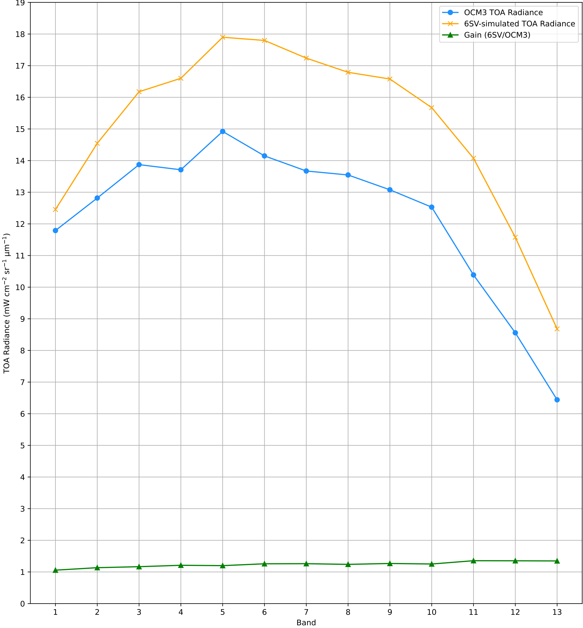
TOA Radiance (OCM3 vs. 6SV) over RVUS RadCalNet Site Lat: 38.497°, Lon: -115.69° - 19-AUG-2025 (STRIP_ID: 14427)
