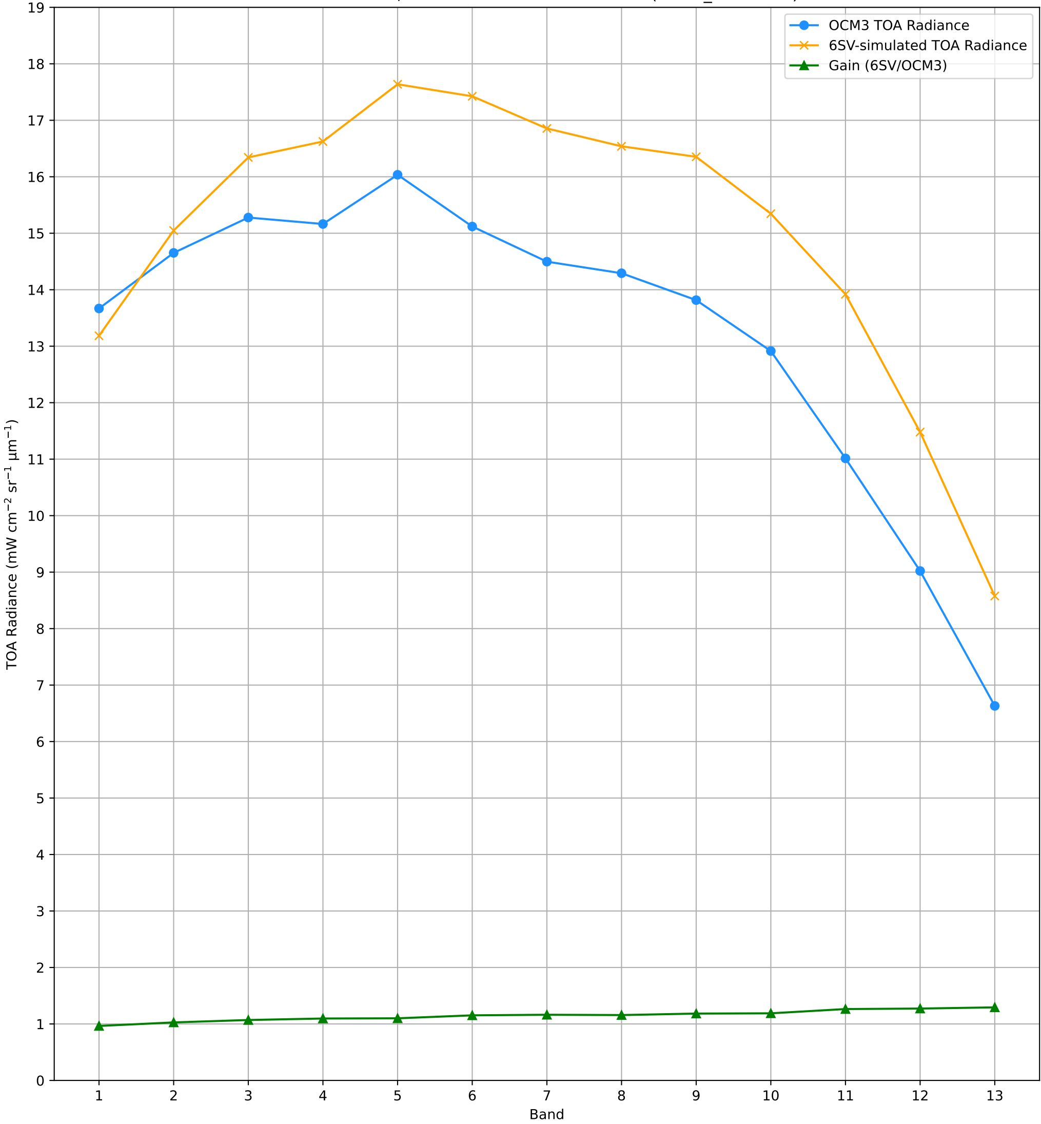
TOA Radiance (OCM3 vs. 6SV) over RVUS RadCalNet Site Lat: 38.497°, Lon: -115.69° - 24-AUG-2025 (STRIP_ID: 14499)
